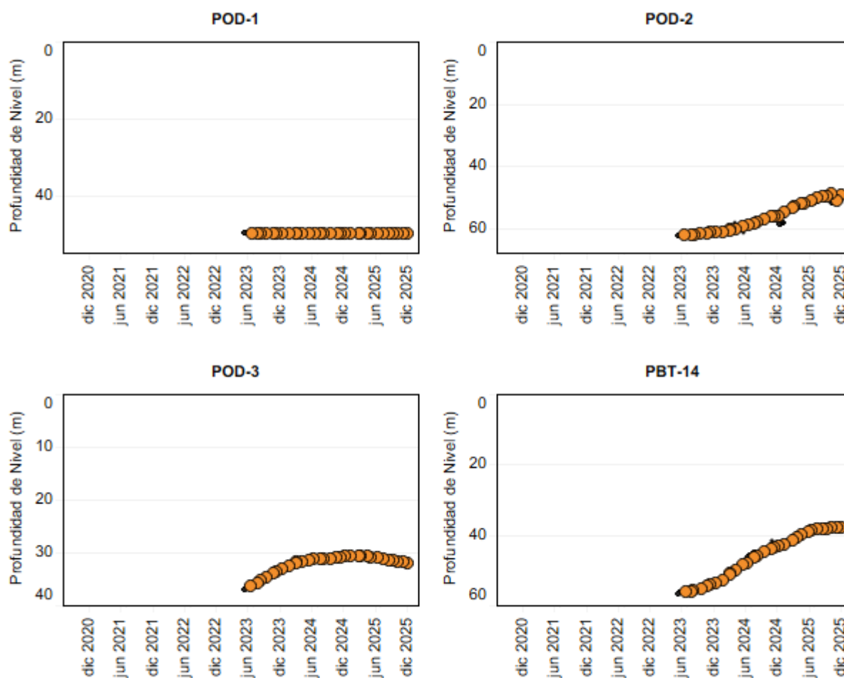
Figura 5-30: Registro continuo de la profundidad de nivel de agua en los puntos asociados al nuevo campo de pozos PBT-14, POD-1, POD-2 y POD-3.
