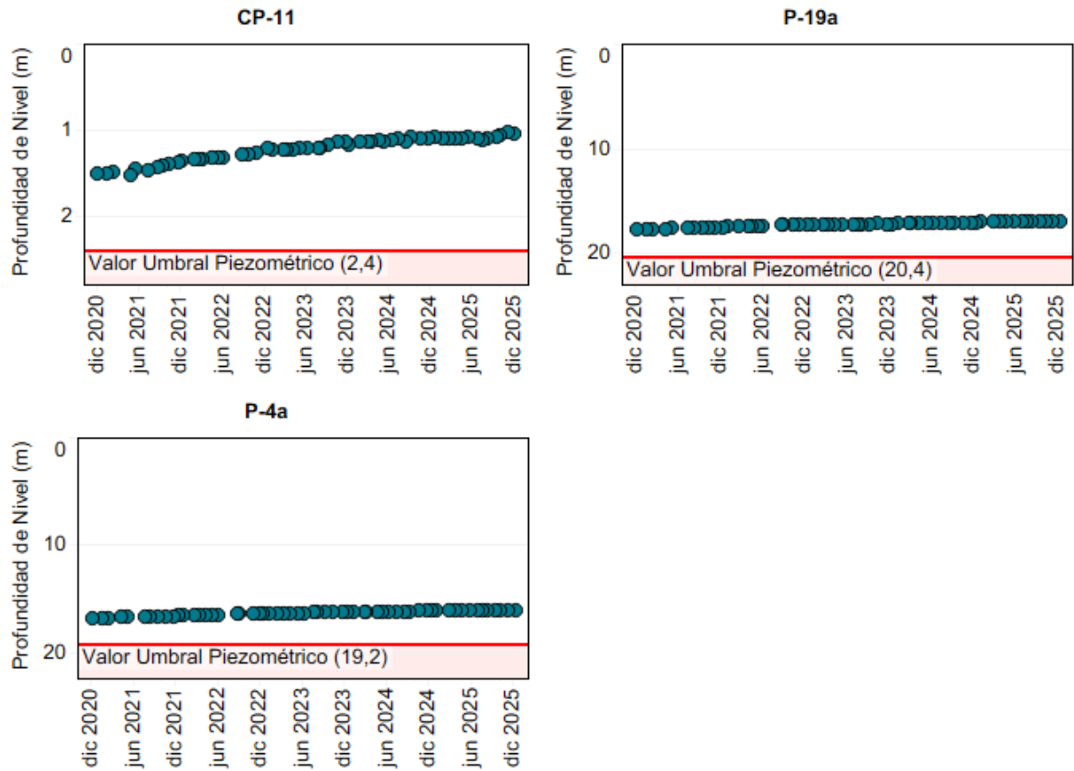
Figura 5-15: Profundidad de nivel en el punto de control CP-11, P-19a y P-4a.
