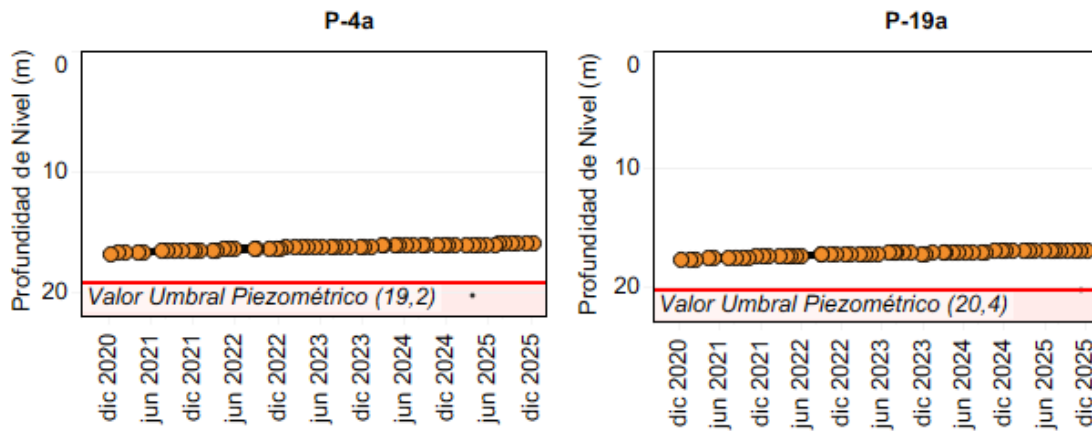
Figura 5-28: Registro continuo de la profundidad de nivel de agua en los puntos de control/avenimiento P-4a y P-19a.
