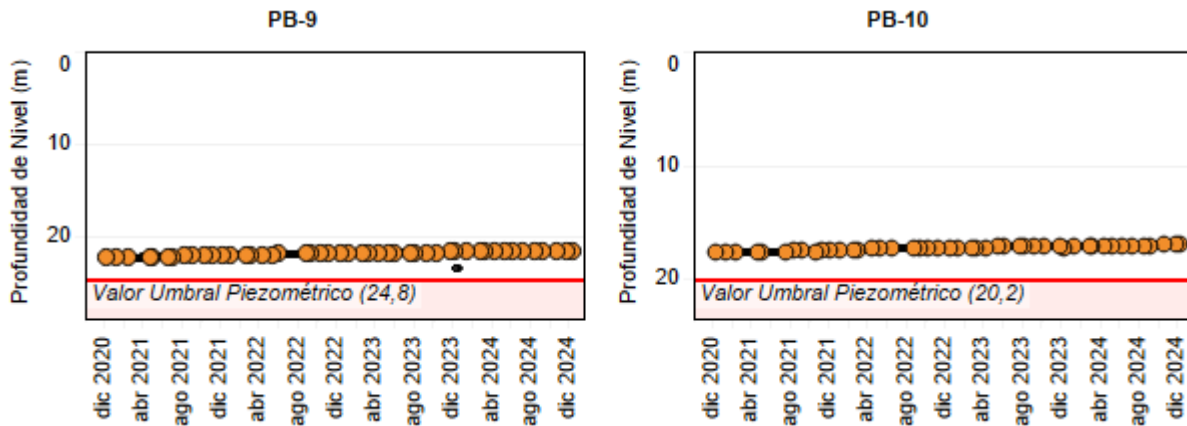
Figura 5-22: Registro continuo de la profundidad de nivel en los puntos de seguimiento PB-9 y PB-10.
