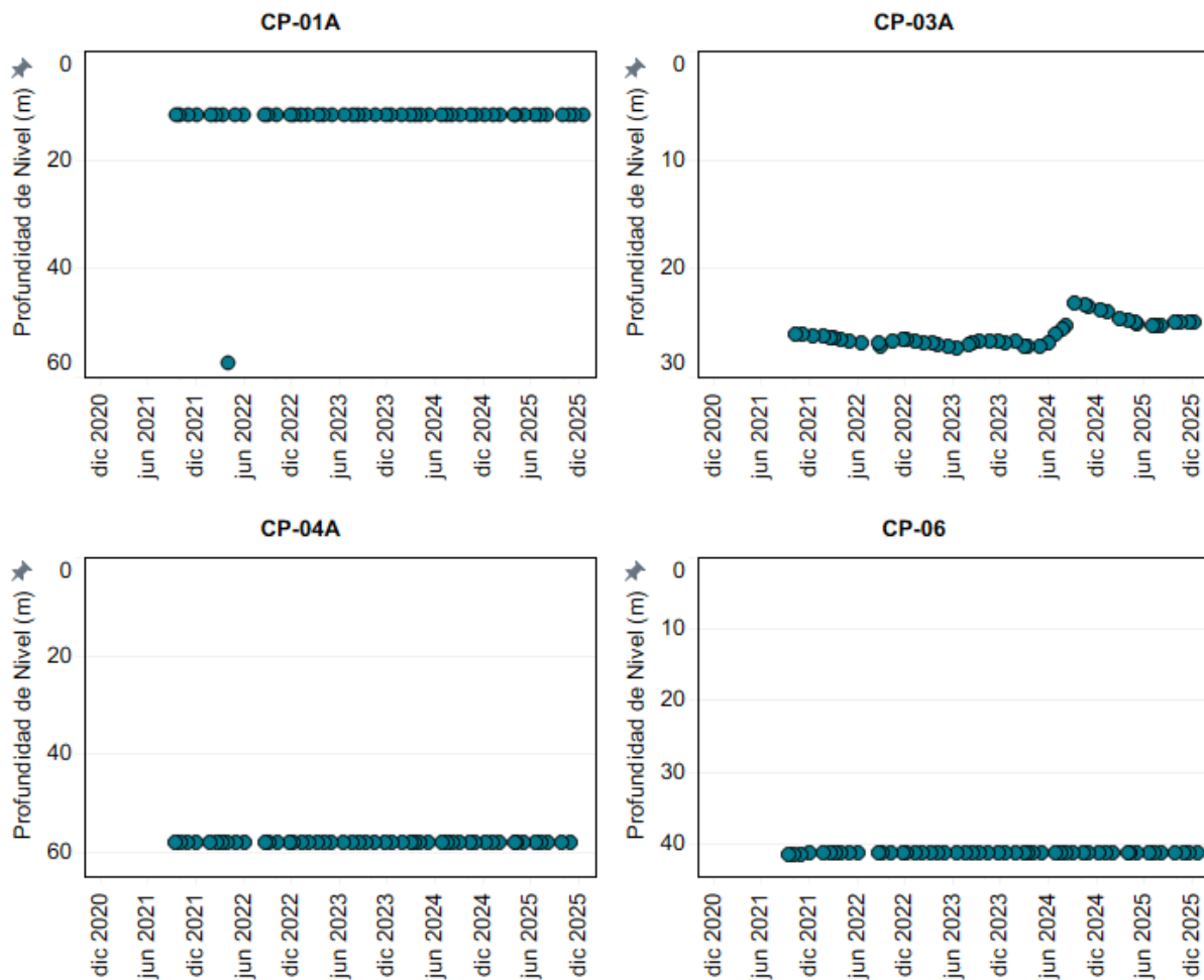
Figura 5-9: Profundidad de nivel de agua en los puntos de monitoreo por Avenimiento CP-01A, CP-03A; CP-04A y CP-06.
