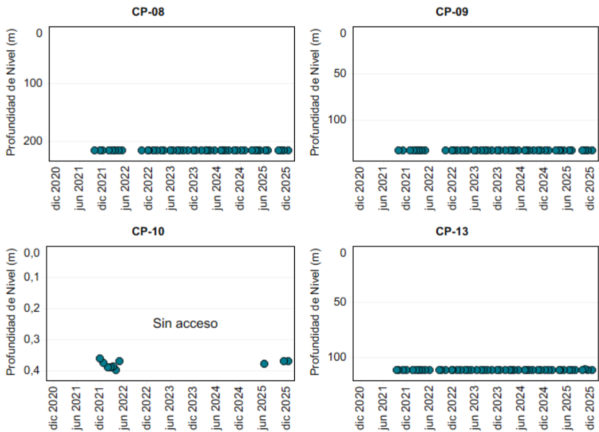
Figura 5-10: Profundidad de nivel de agua en los puntos de monitoreo por Avenimiento CP-08, CP-09; CP-10 y CP-13.
