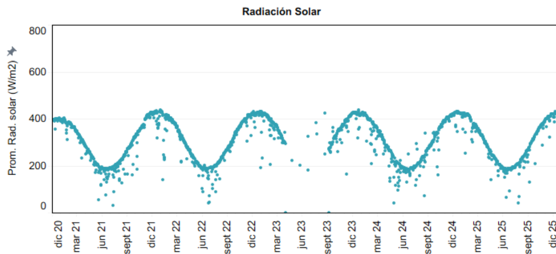
Figura 4-18: Radiación solar media diaria en estación La Ola.
