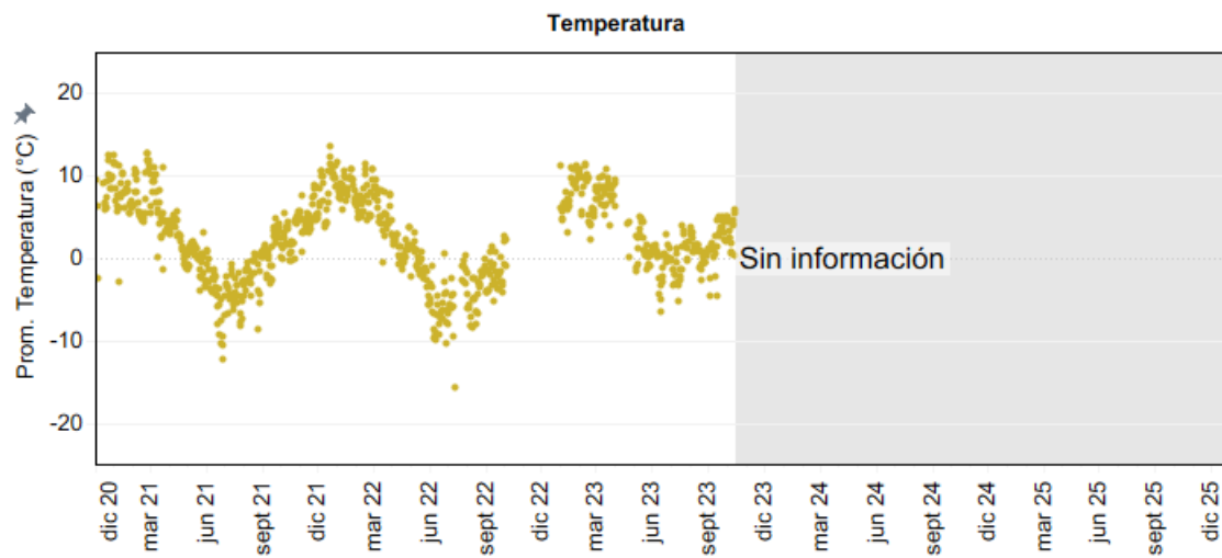
Figura 4-10: Temperatura ambiental media diaria en estación Los Arroyos.
