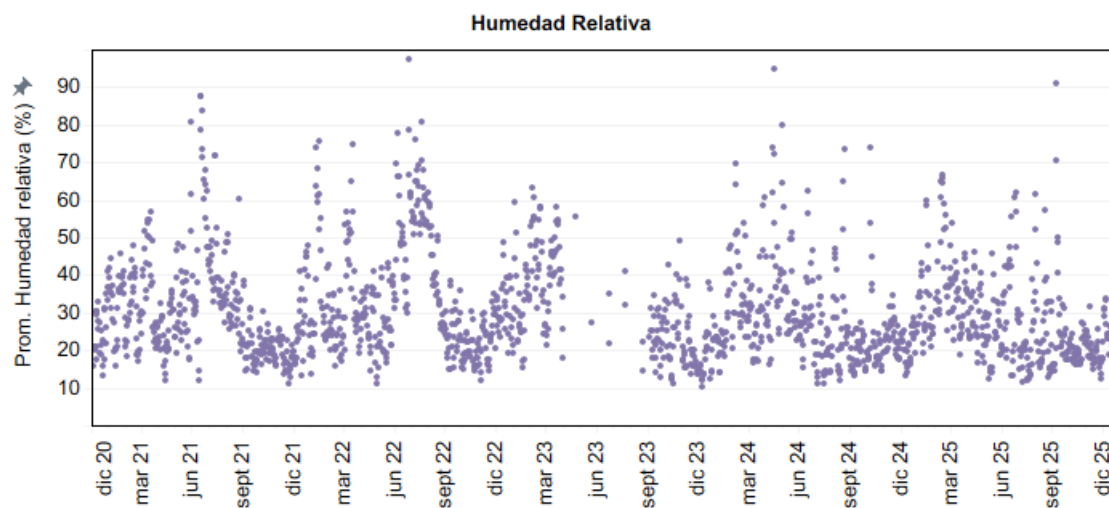
Figura 4-12: Humedad relativa media diaria en estación La Ola.
