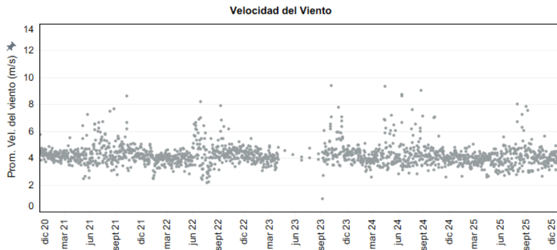
Figura 4-6: Velocidad media diaria en estación La Ola.
