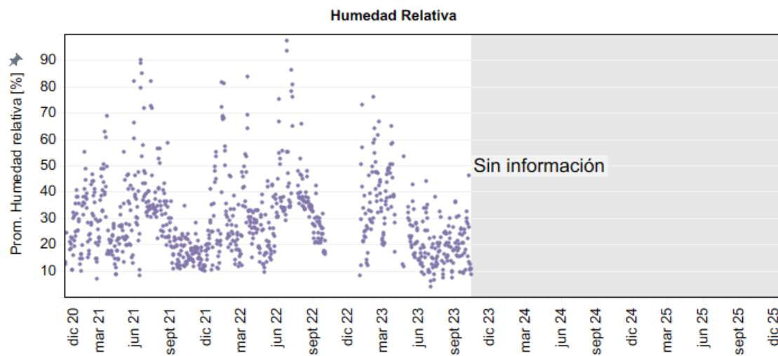
Figura 4-13: Humedad relativa media diaria en estación Los Arroyos.
