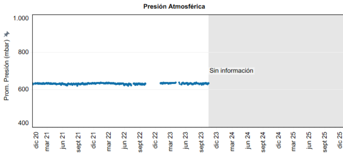
Figura 4-16: Presión atmosférica media diaria en estación Los Arroyos.
