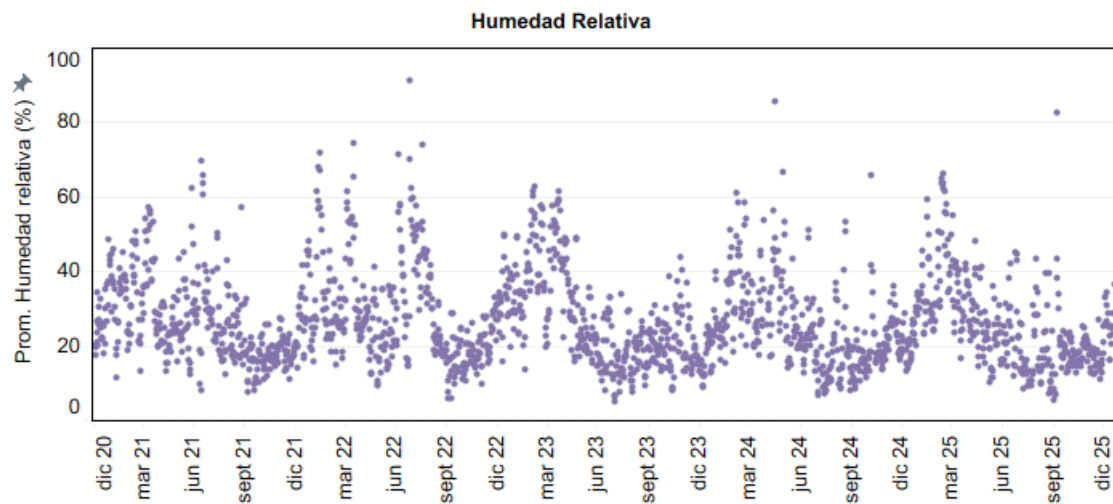
Figura 4-14: Humedad relativa media diaria en estación Centro Salar
