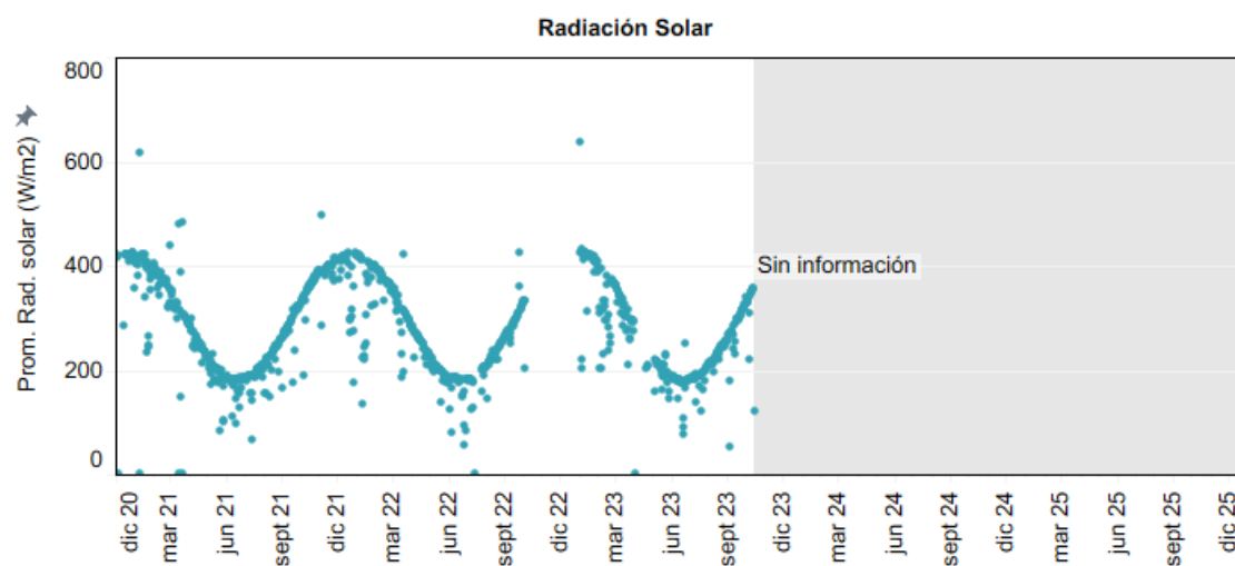
Figura 4-19: Radiación solar media diaria en estación Los Arroyos.
