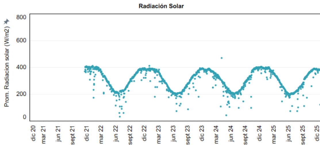
Figura 4-20: Radiación solar media diaria en estación Centro Salar.
