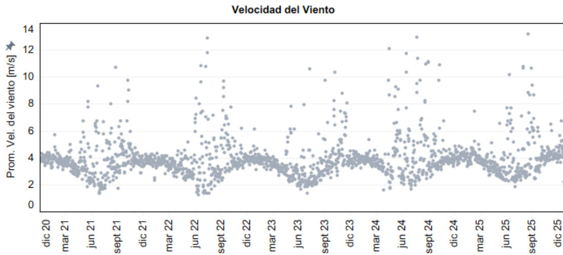
Figura 4-8: Velocidad media diaria en estación Centro Salar.
