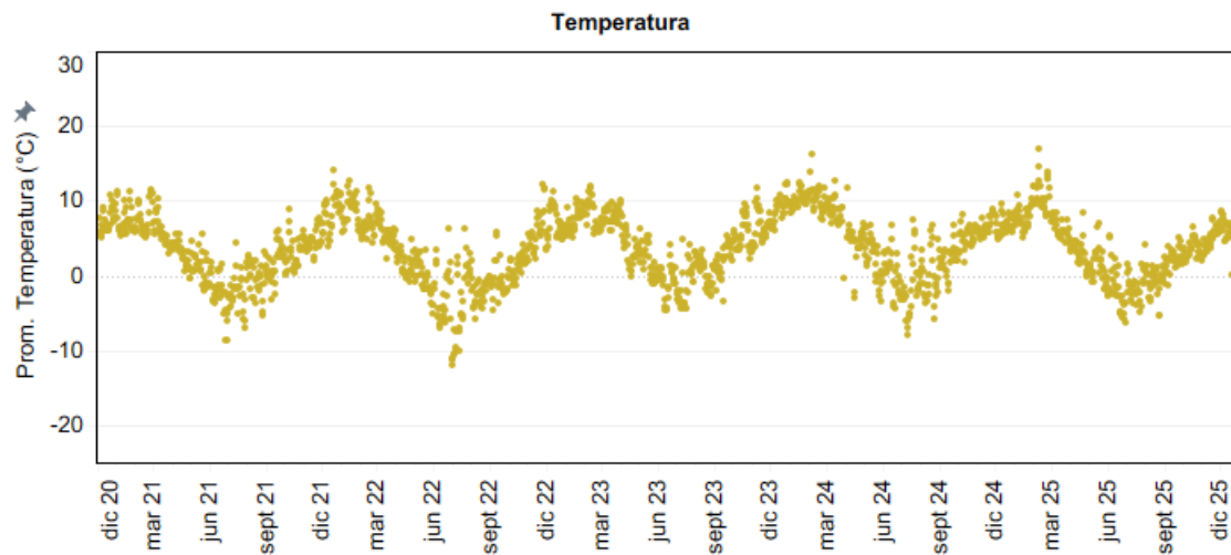
Figura 4-11: Temperatura ambiental media diaria en estación Centro Salar.
