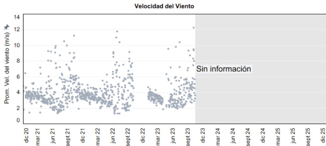
Figura 4-7: Velocidad media diaria en estación Los Arroyos.
