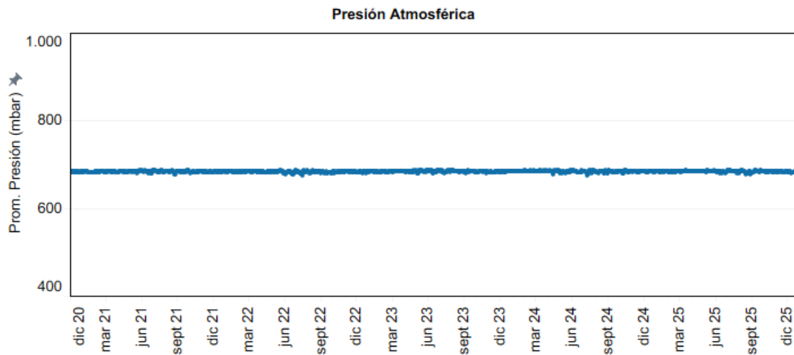
Figura 4-17: Presión atmosférica media diaria en estación Centro Salar.
