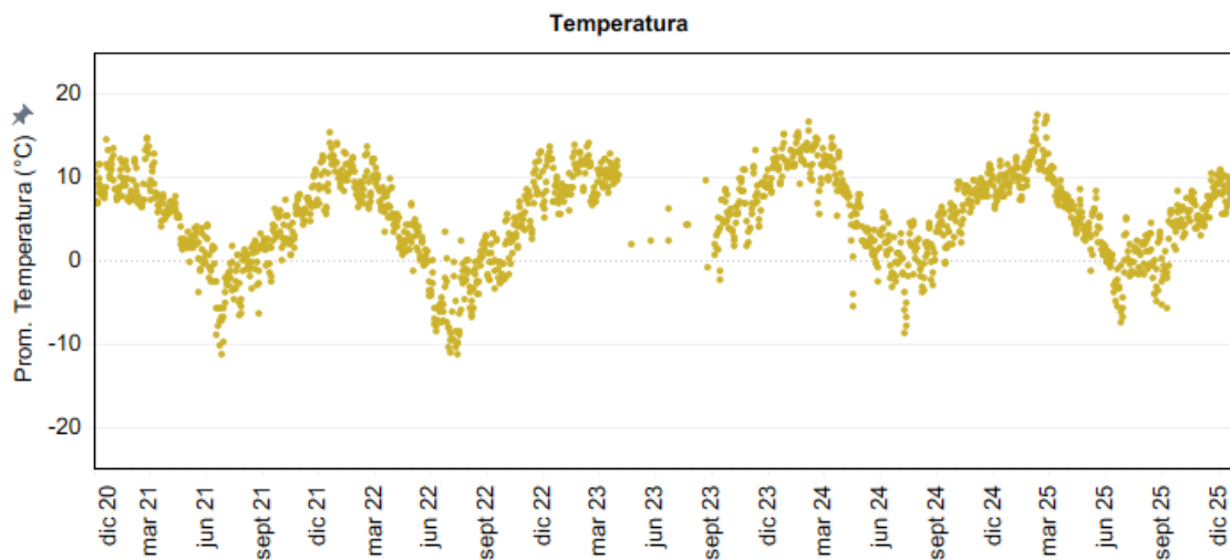
Figura 4-9: Temperatura ambiental media diaria en estación La Ola.
