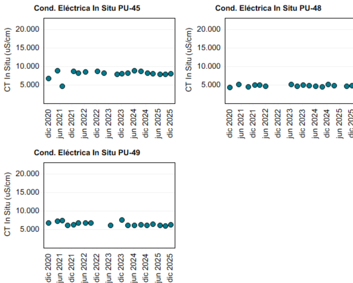
Figura 4-10. Evolución temporal de Conductividad eléctrica in situ ( \mu\text{S/cm} ) en los puntos PU-45, PU-48 y PU-49.
