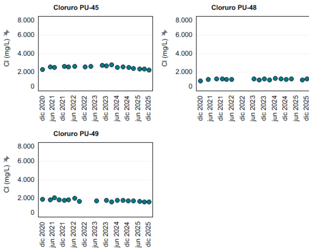
Figura 4-68: Evolución temporal de Cloruro (mg/L) en los puntos PU-45, PU-48 y PU-49.
