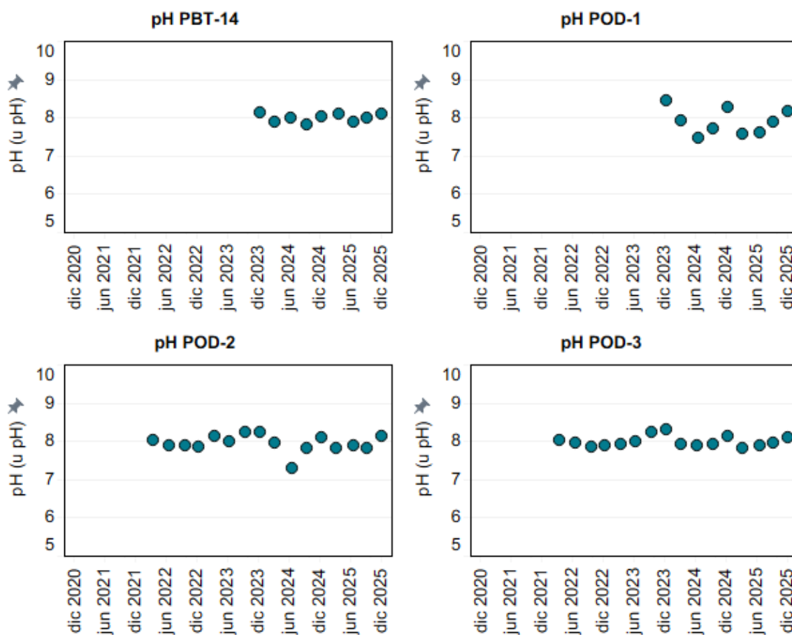
Figura 4-20: Evolución temporal de pH (unidades de pH) en los puntos PBT-14, POD-1, POD-2 y POD-3.
