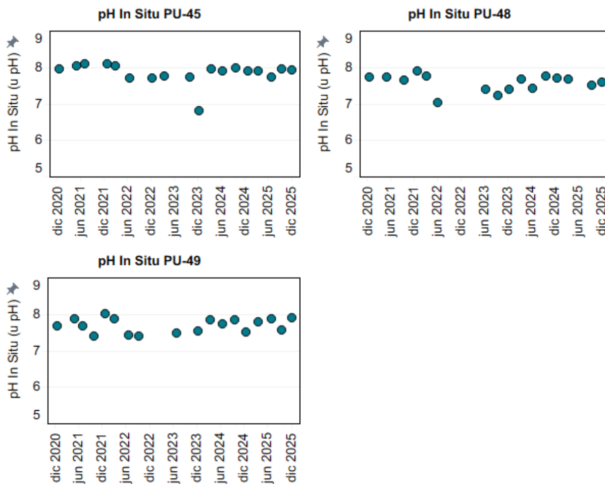
Figura 4-12: Evolución temporal de pH in situ (unidades de pH) en los puntos PU-45, PU-48 y PU-49.
