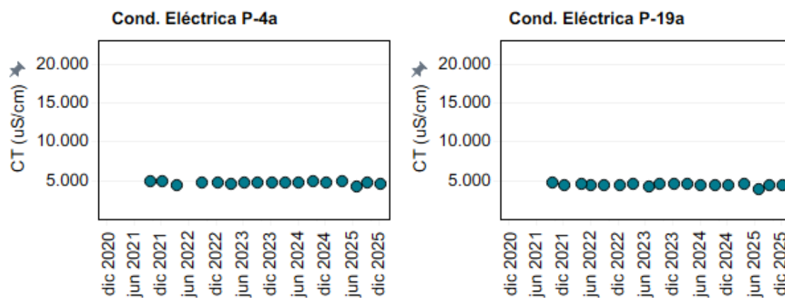
Figura 4-14: Evolución temporal de Conductividad eléctrica ( \mu\text{S}/\text{cm} ) en los puntos P-4a y P-19a.
