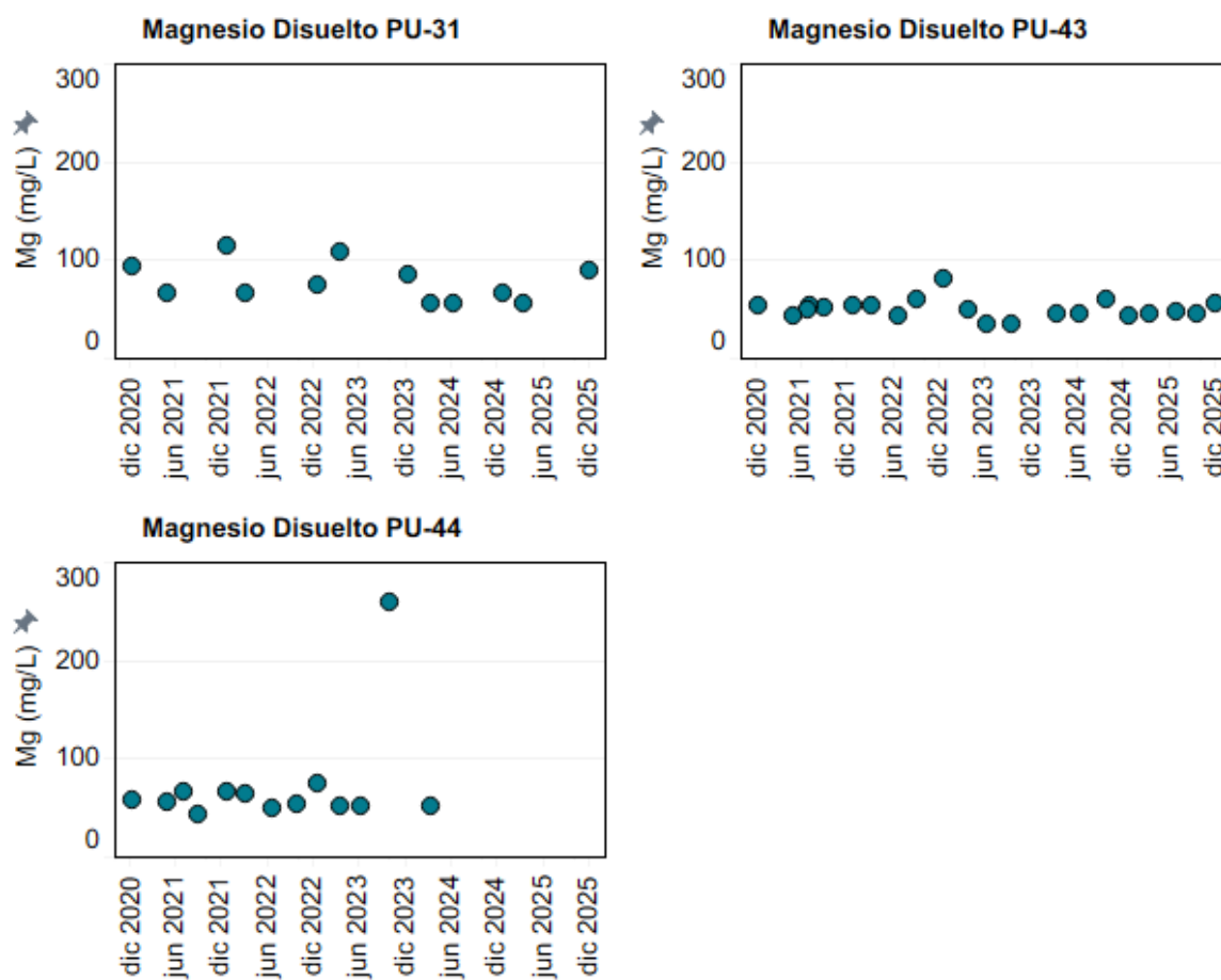
Figura 4-59: Evolución temporal de Magnesio disuelto (mg/L) en los puntos PU-31, PU-43 y PU-44.
