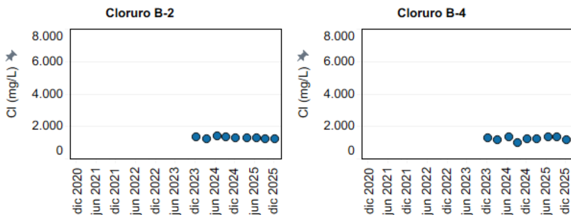
Figura 4-47: Evolución temporal de Cloruro (mg/L) en los puntos B-2 y B-4.
