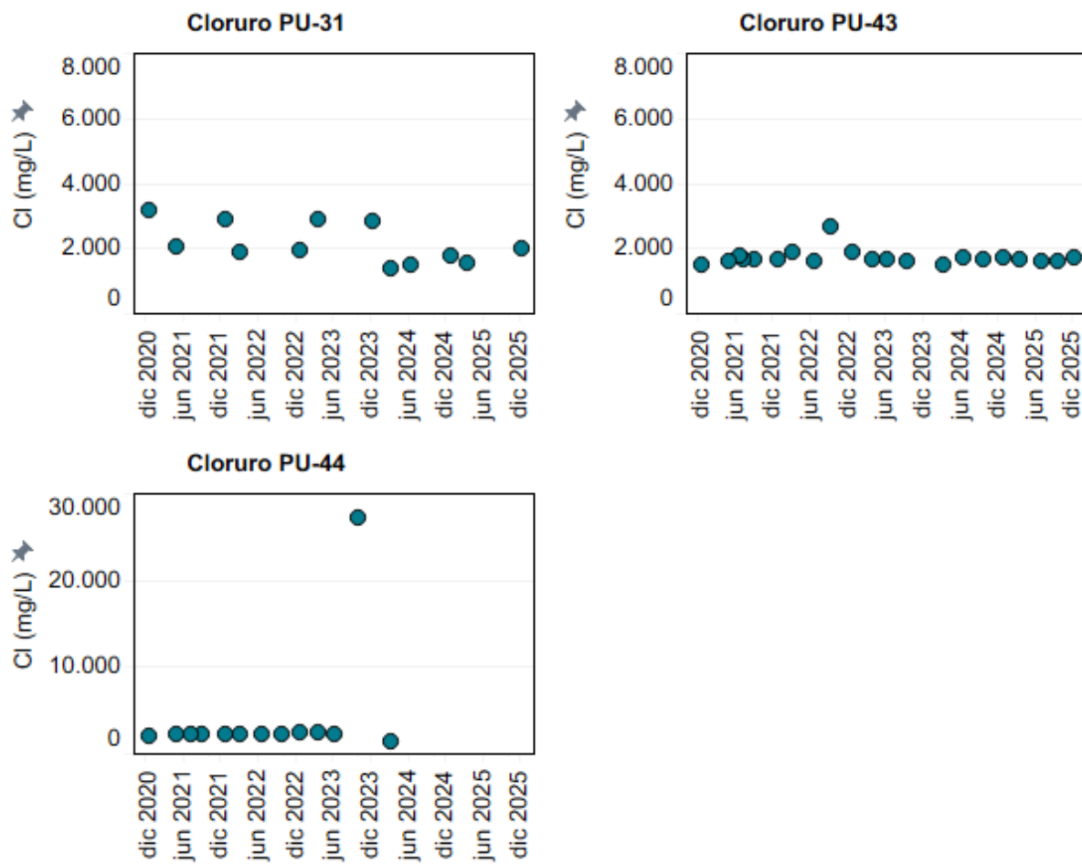
Figura 4-67: Evolución temporal de Cloruro (mg/L) en los puntos PU-31, PU-43 y PU-44.
