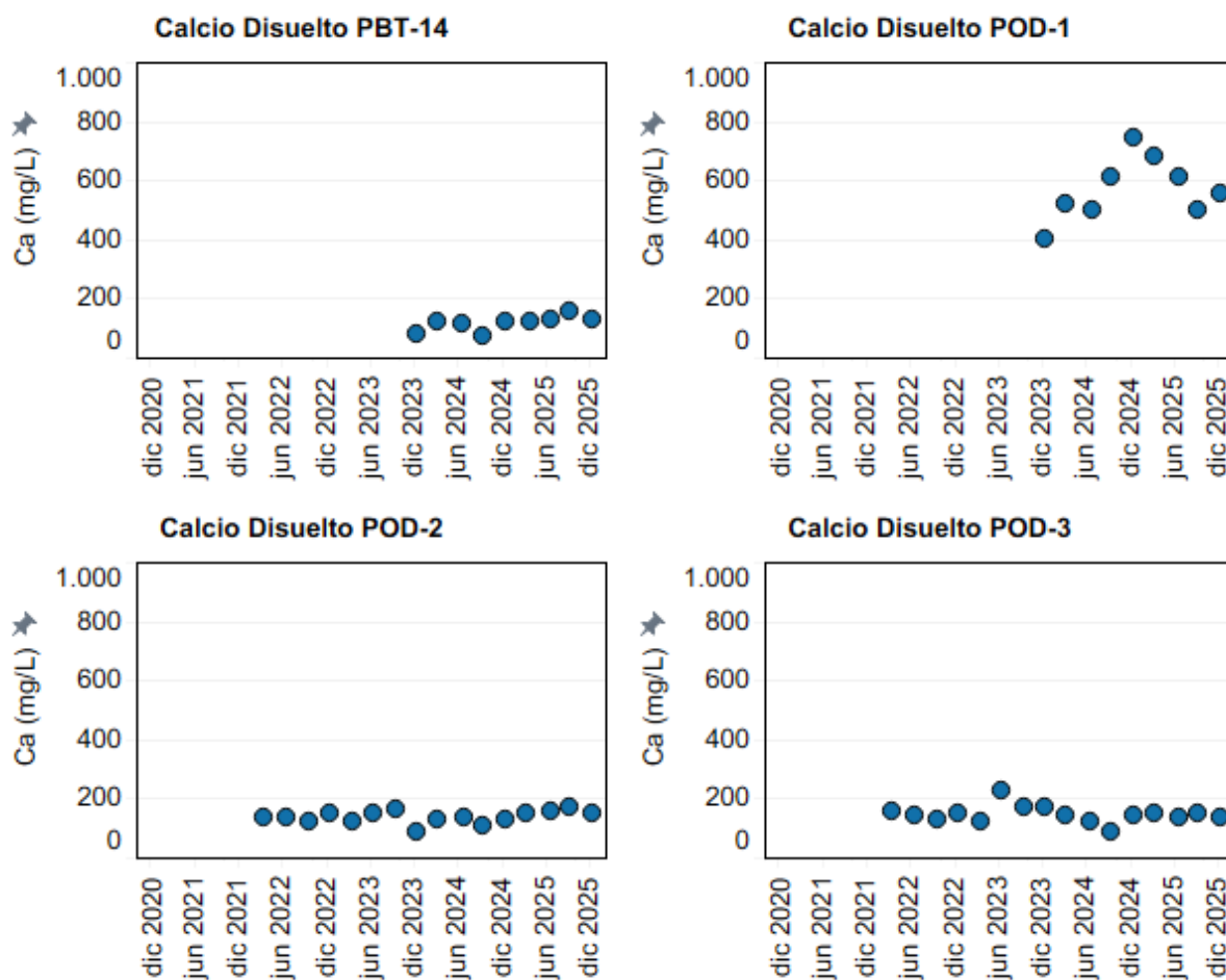
Figura 4-28: Evolución temporal de Calcio disuelto (mg/L) en los puntos PBT-14, POD-1, POD-2 y POD-3.
