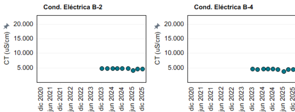
Figura 4-15: Evolución temporal de Conductividad eléctrica ( \mu\text{S/cm} ) en los puntos B-2 y B-4.
