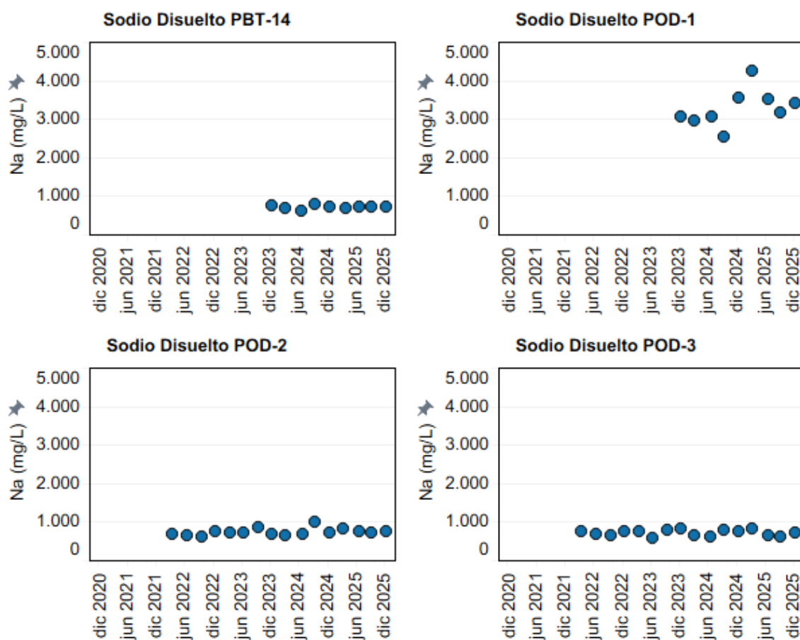
Figura 4-40: Evolución temporal de Sodio disuelto (mg/L) en los puntos PBT-14, POD-1, POD-2 y POD-3.
