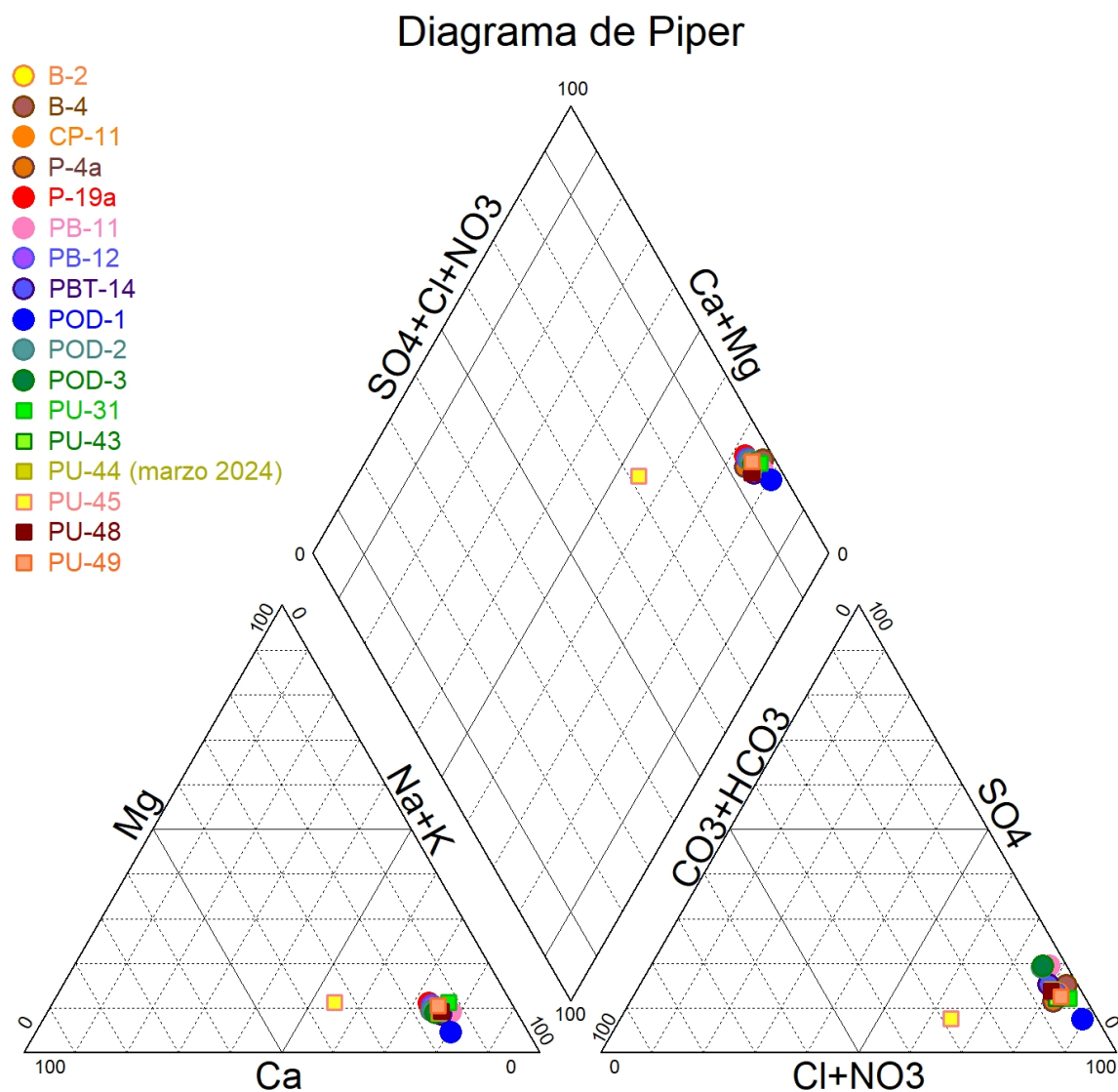
Figura 5-10: Diagrama Piper de los puntos monitoreados en el segundo semestre 2025.
