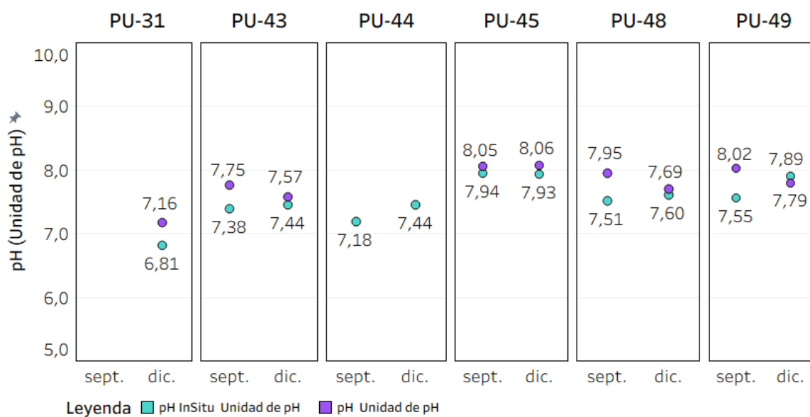
Figura 5-8: Comparación entre el pH medido in situ y laboratorio en las punteras PU-31, PU-43, PU-44, PU-45, PU-48 y PU-49.
