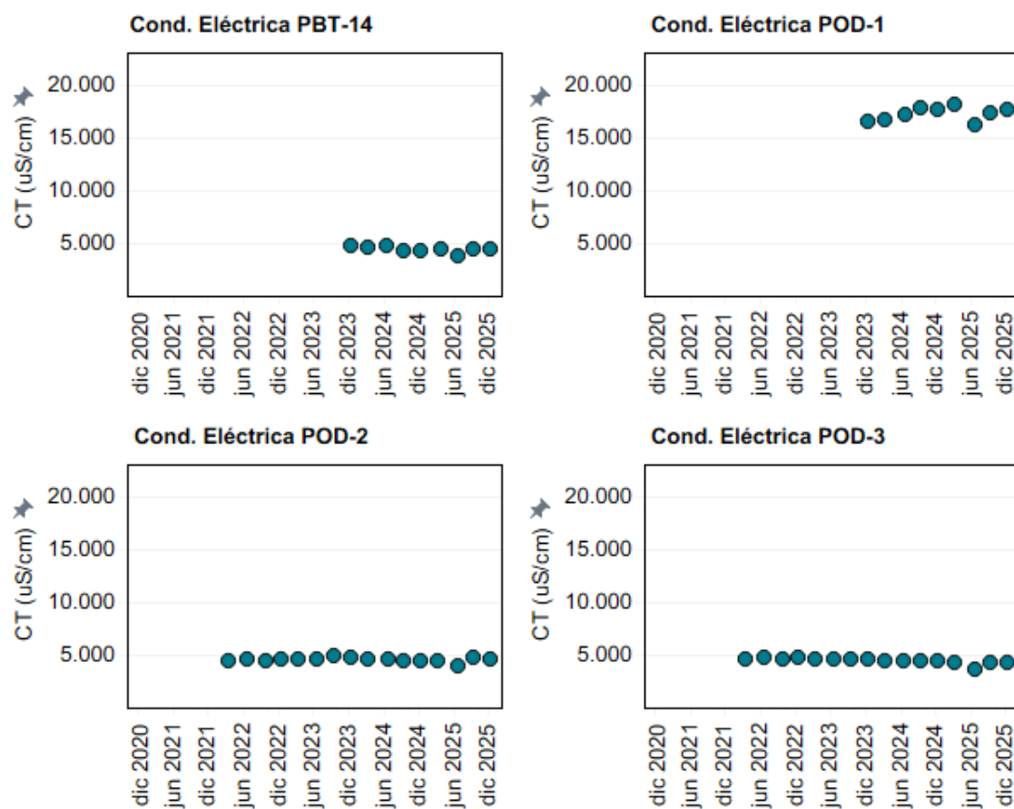
Figura 4-16: Evolución temporal de Conductividad eléctrica ( \mu\text{S/cm} ) en los puntos PBT-14, POD-1, POD-2 y POD-3.
