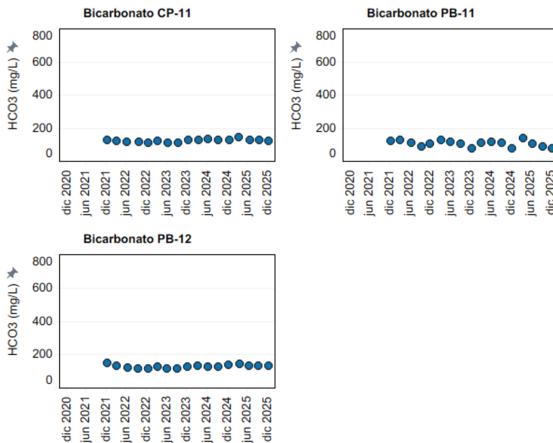
Figura 4-41: Evolución temporal de Bicarbonato (mg/L) en los puntos CP-11, PB-11 y PB-12.
