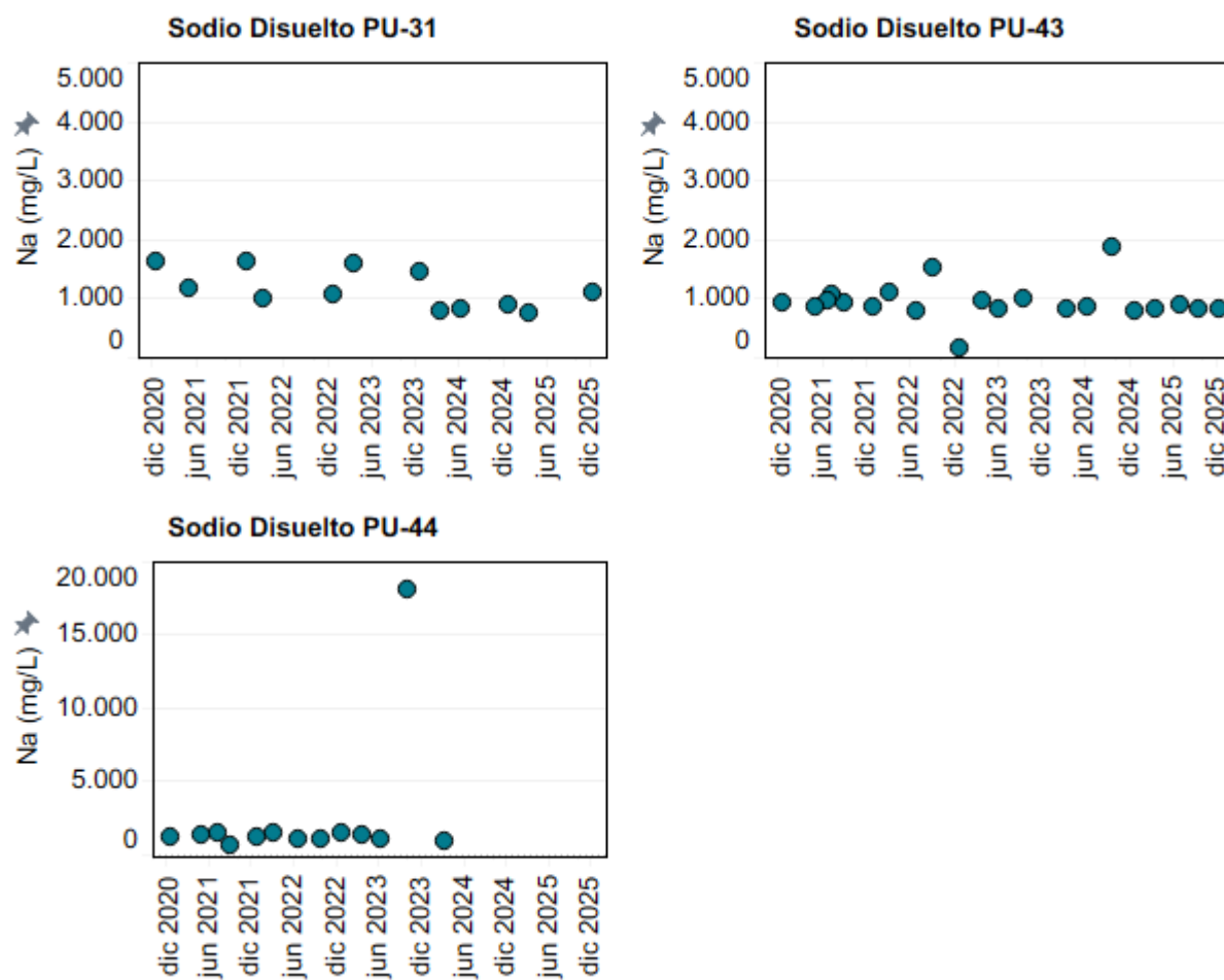
Figura 4-63: Evolución temporal de Sodio disuelto (mg/L) en los puntos PU-31, PU-43 y PU-44.
