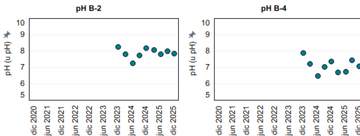
Figura 4-19: Evolución temporal de pH (unidades de pH) en los puntos B-2 y B-4.
