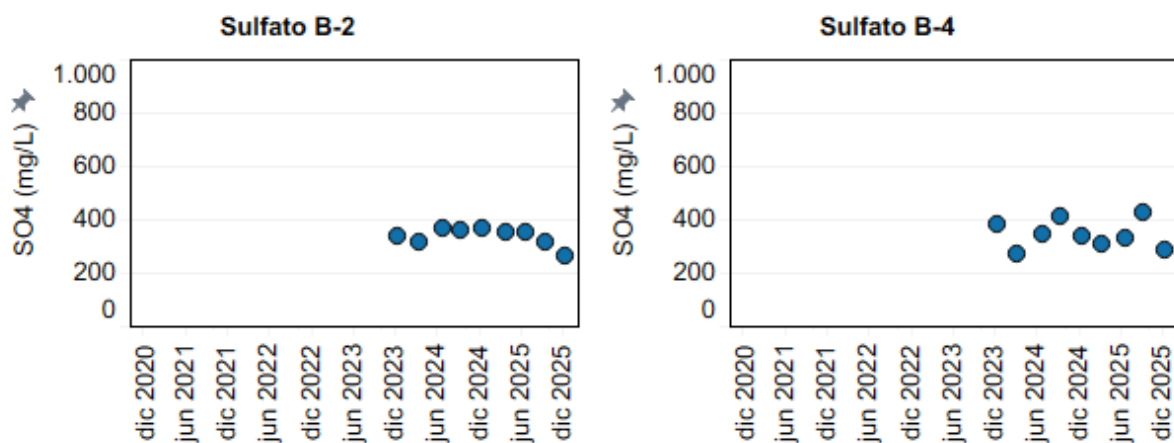
Figura 4-55: Evolución temporal de Sulfato (mg/L) en los puntos B-2 y B-4.
