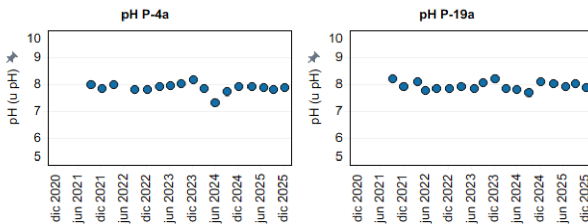
Figura 4-18: Evolución temporal de pH (unidades de pH) en los puntos P-4a y P-19a.
