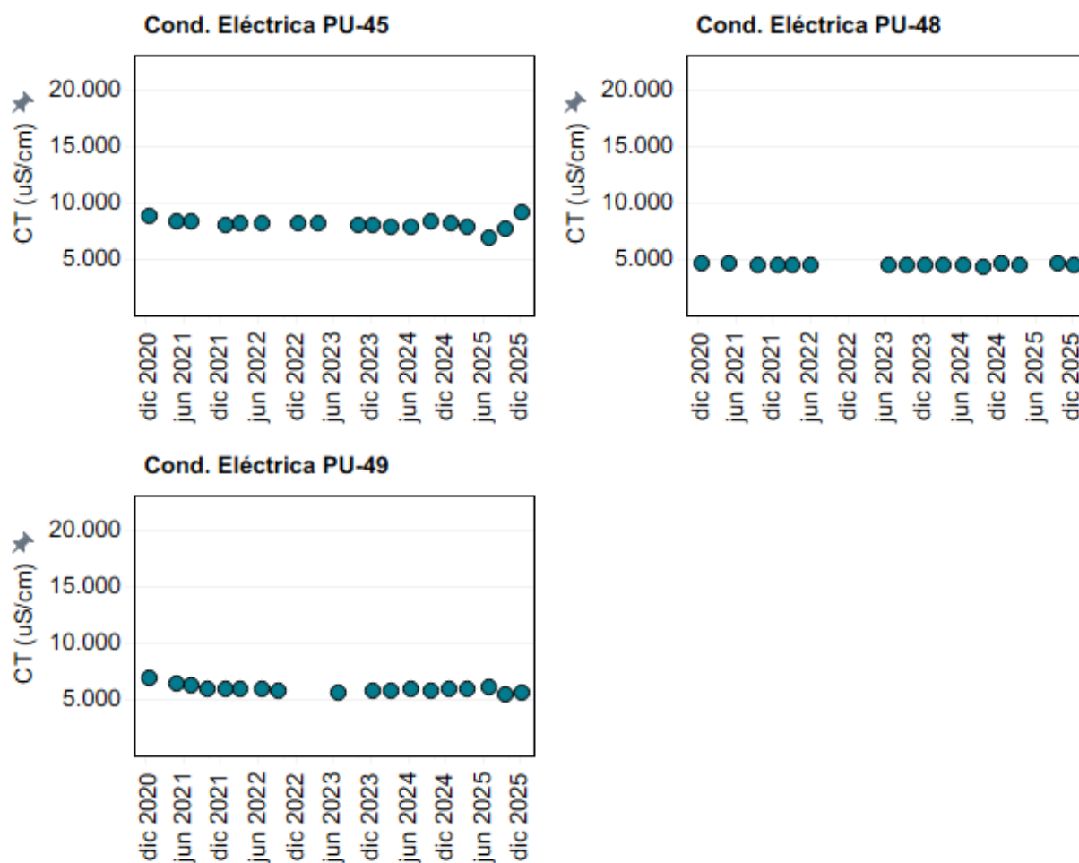
Figura 4-22: Evolución temporal de Conductividad eléctrica ( \mu\text{S}/\text{cm} ) en los puntos PU-45, PU-48 y PU-49.
