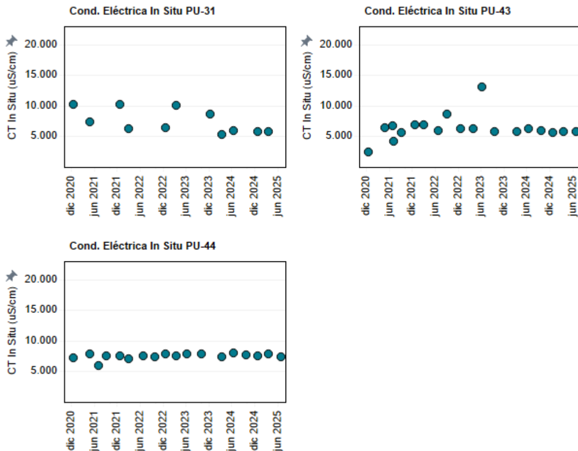
Figura 4-9. Evolución temporal de Conductividad eléctrica in situ ( \mu\text{S}/\text{cm} ) en los puntos PU-31, PU-43 y PU-44.
