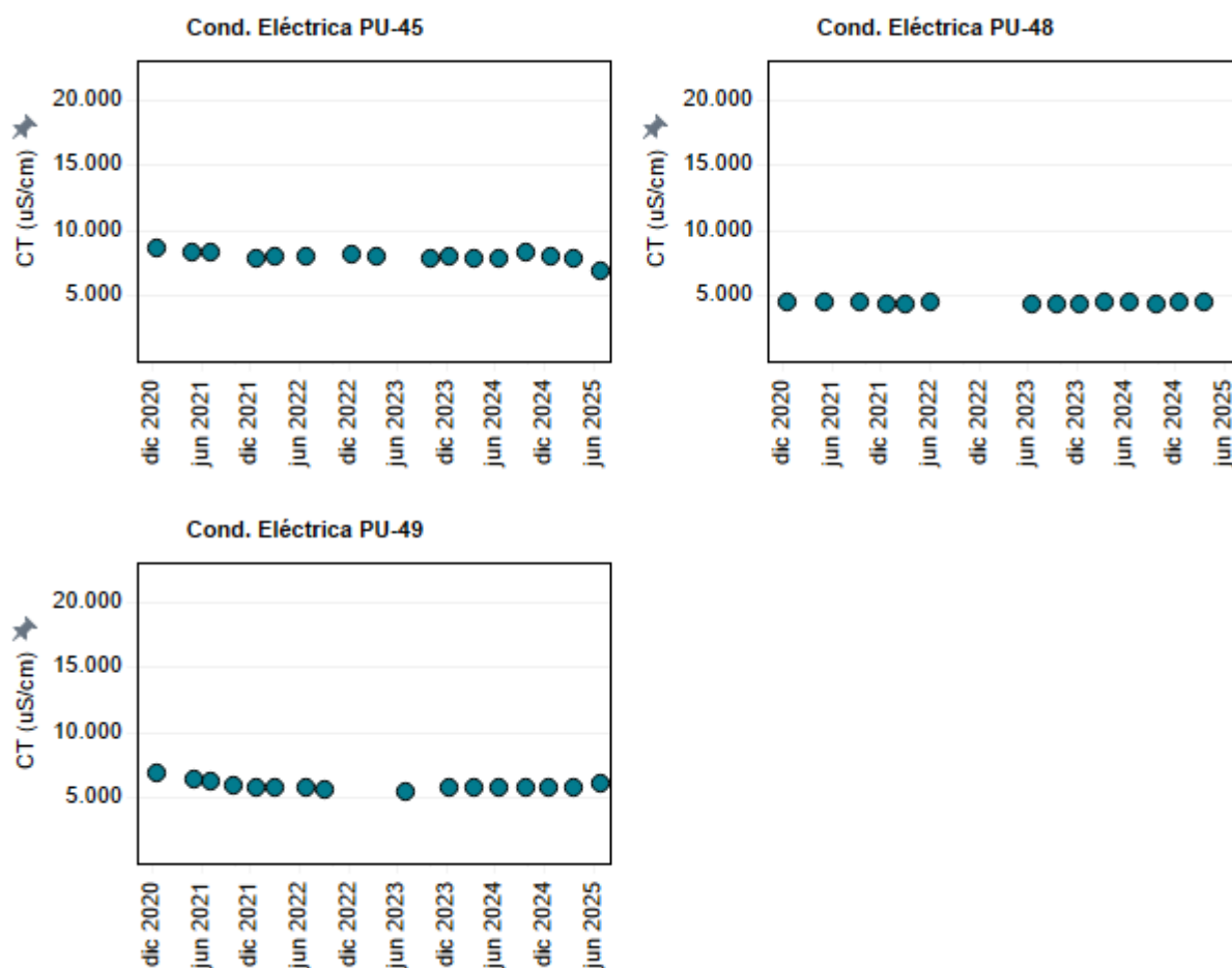
Figura 4-22: Evolución temporal de Conductividad eléctrica ( \mu\text{S/cm} ) en los puntos PU-45, PU-48 y PU-49.
