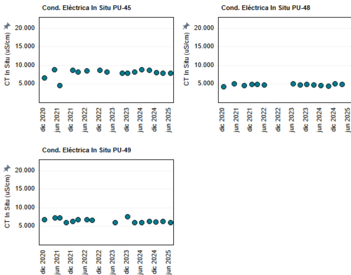
Figura 4-10. Evolución temporal de Conductividad eléctrica in situ ( \mu\text{S/cm} ) en los puntos PU-45, PU-48 y PU-49.
