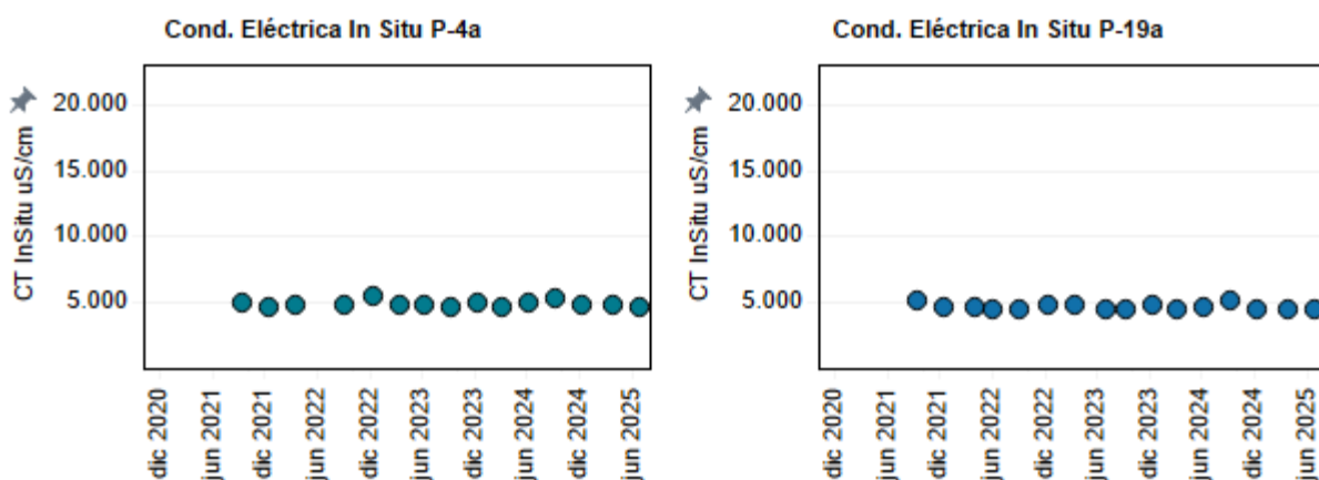
Figura 4-2: Evolución temporal de Conductividad eléctrica in situ ( \mu\text{S/cm} ) en los puntos P-4a y P-19a.
