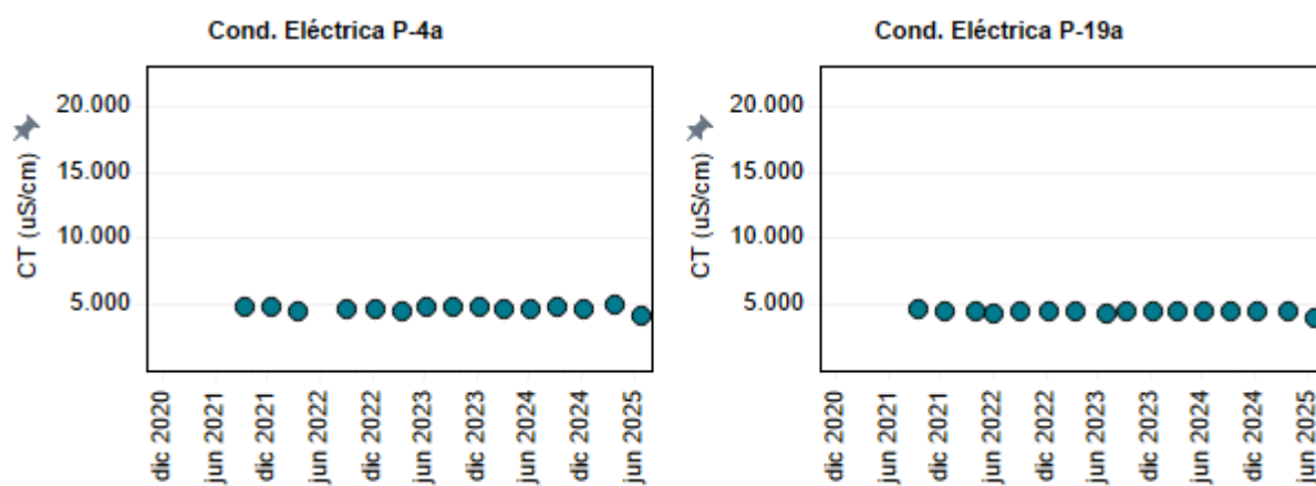
Figura 4-14: Evolución temporal de Conductividad eléctrica ( \mu\text{S/cm} ) en los puntos P-4a y P-19a.
