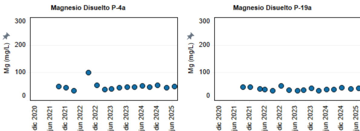
Figura 4-30: Evolución temporal de Magnesio disuelto (mg/L) en los puntos P-4a y P-19a.
