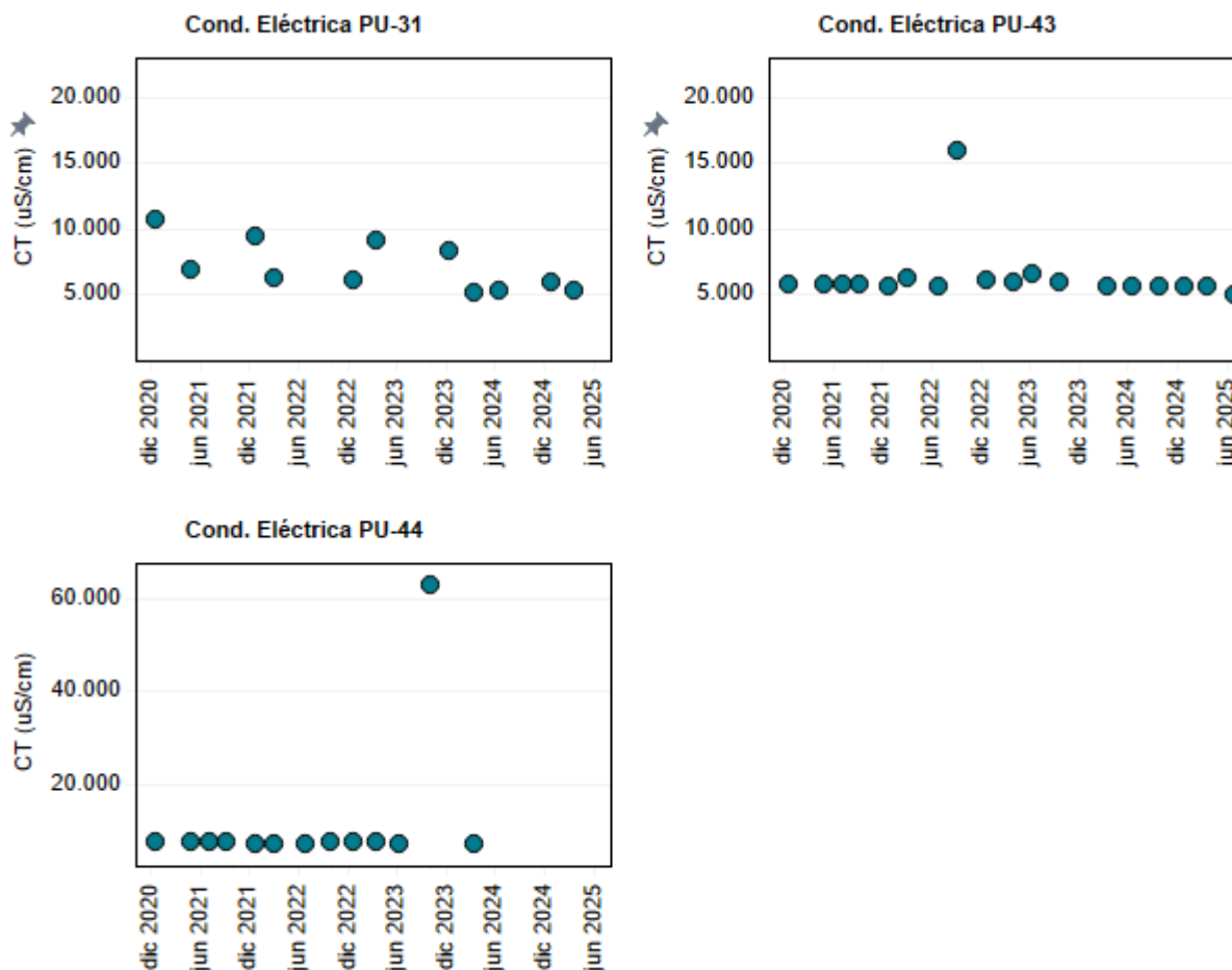
Figura 4-21: Evolución temporal de Conductividad eléctrica ( \mu\text{S}/\text{cm} ) en los puntos PU-31, PU-43 y PU-44.
