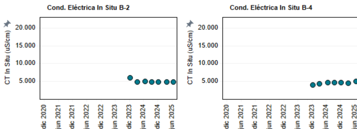
Figura 4-3: Evolución temporal de Conductividad eléctrica in situ ( \mu\text{S/cm} ) en los puntos B-2 y B-4.
