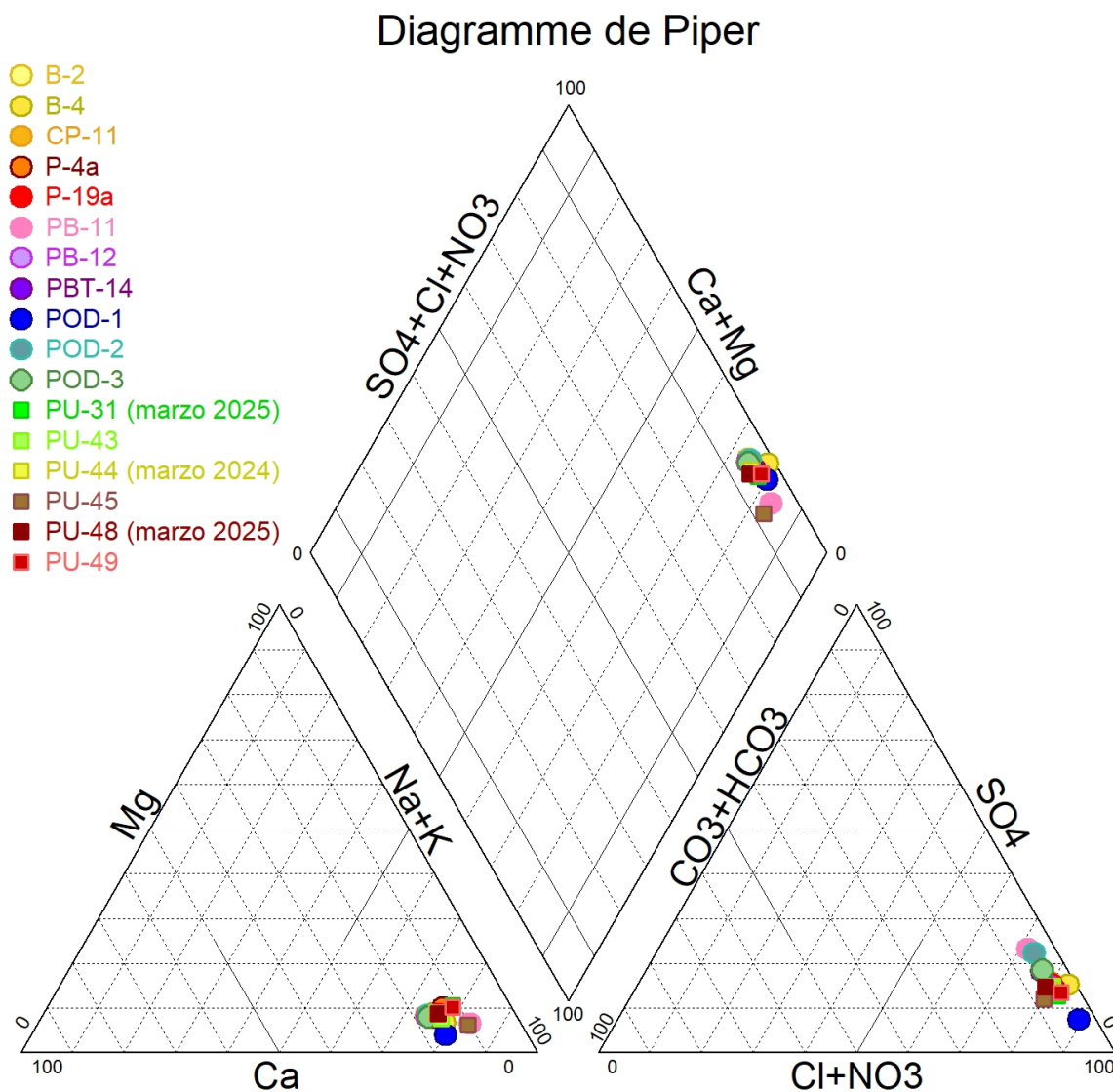
Figura 5-10: Diagrama Piper de los puntos monitoreados en el primer semestre 2025.
