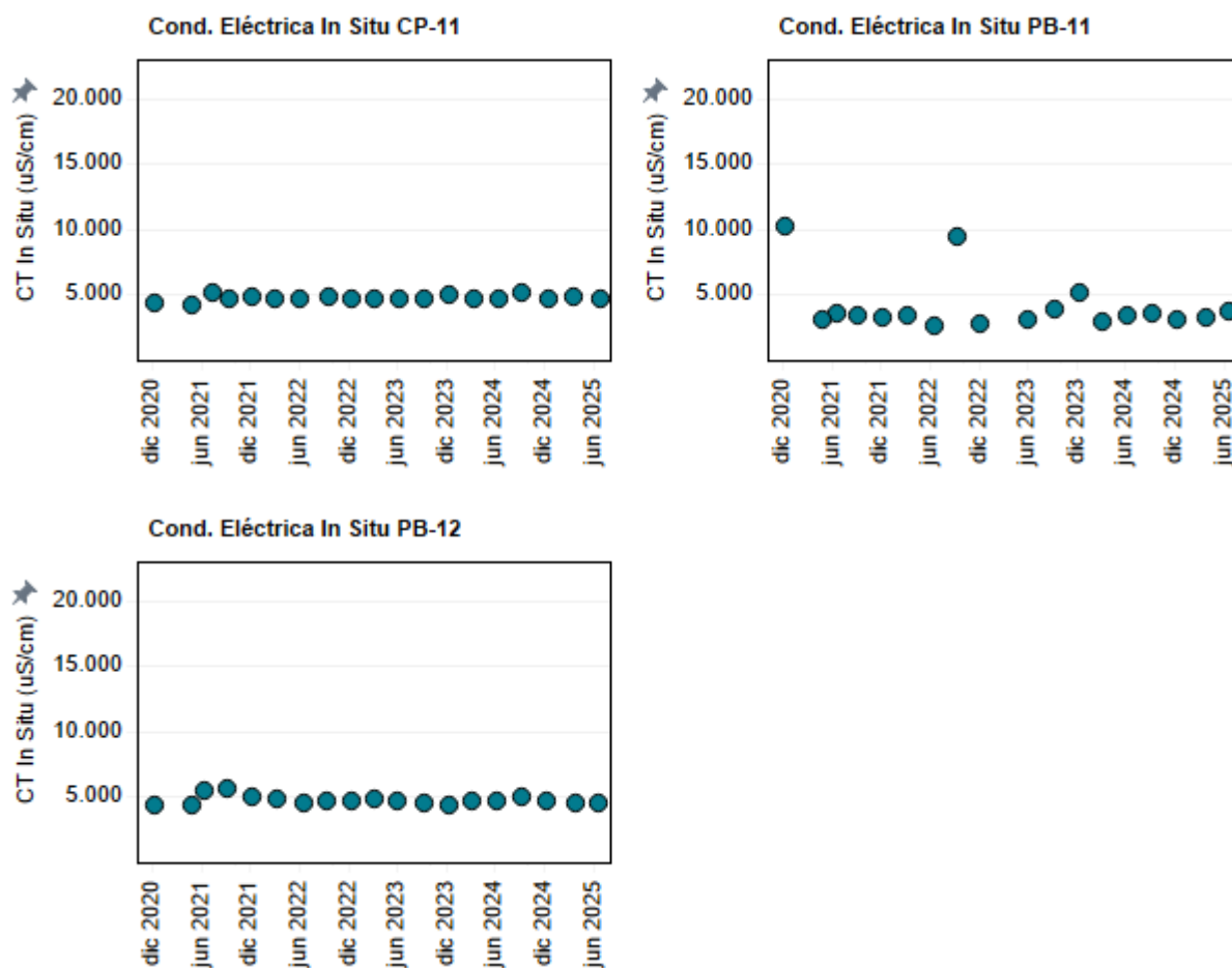
Figura 4-1: Evolución temporal de Conductividad eléctrica in situ ( \mu\text{S/cm} ) en los puntos CP-11, PB-11 y PB-12.
