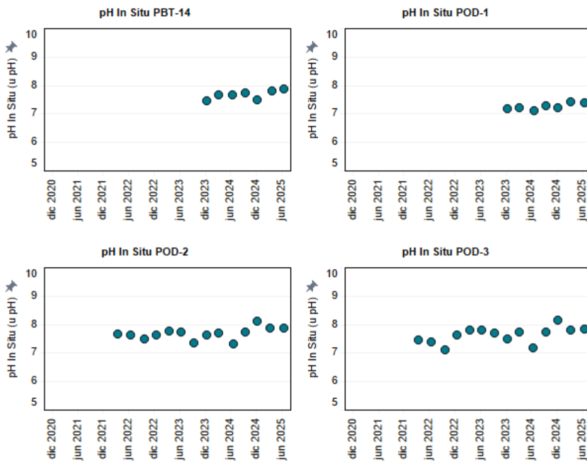
Figura 4-8: Evolución temporal de pH in situ (unidades de pH) en los puntos PBT-14, POD-1, POD-2 y POD-3.
