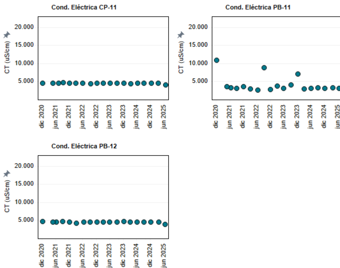
Figura 4-13: Evolución temporal de Conductividad eléctrica ( \mu\text{S/cm} ) en los puntos CP-11, PB-11 y PB-12.
