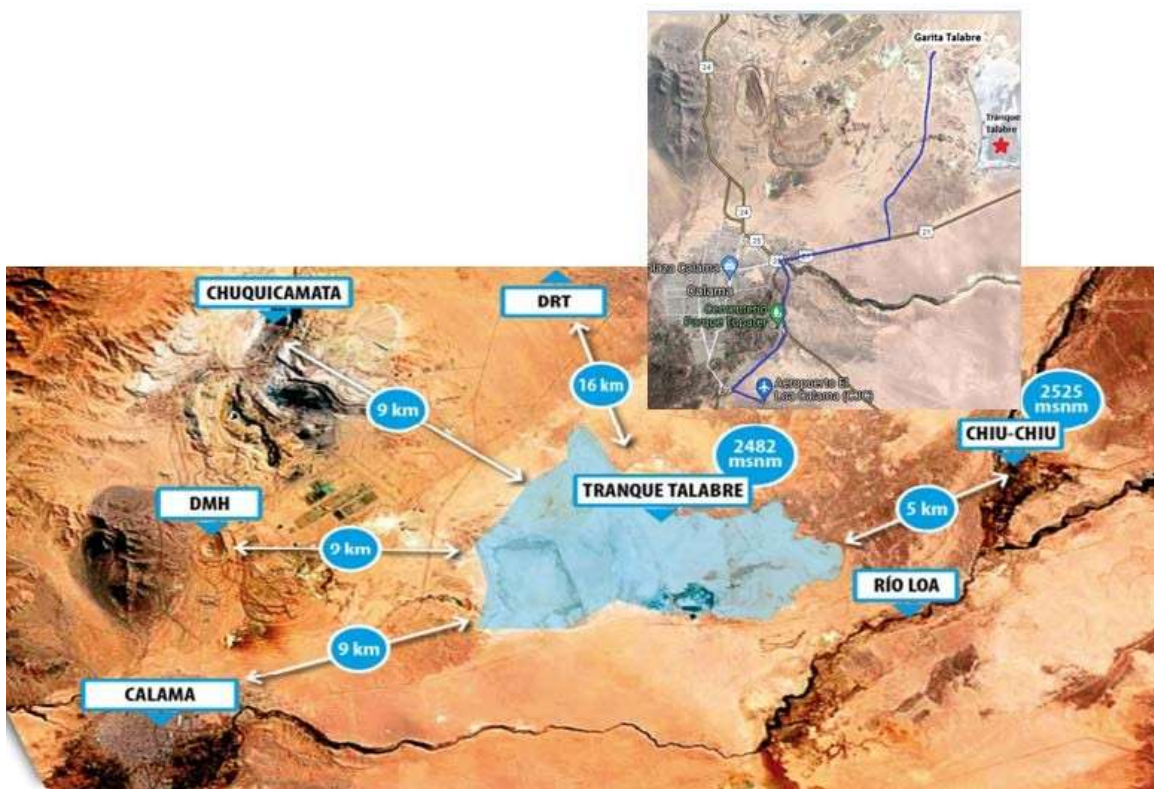
Figura N° 3 Ubicación y acceso Tranque Talabre
