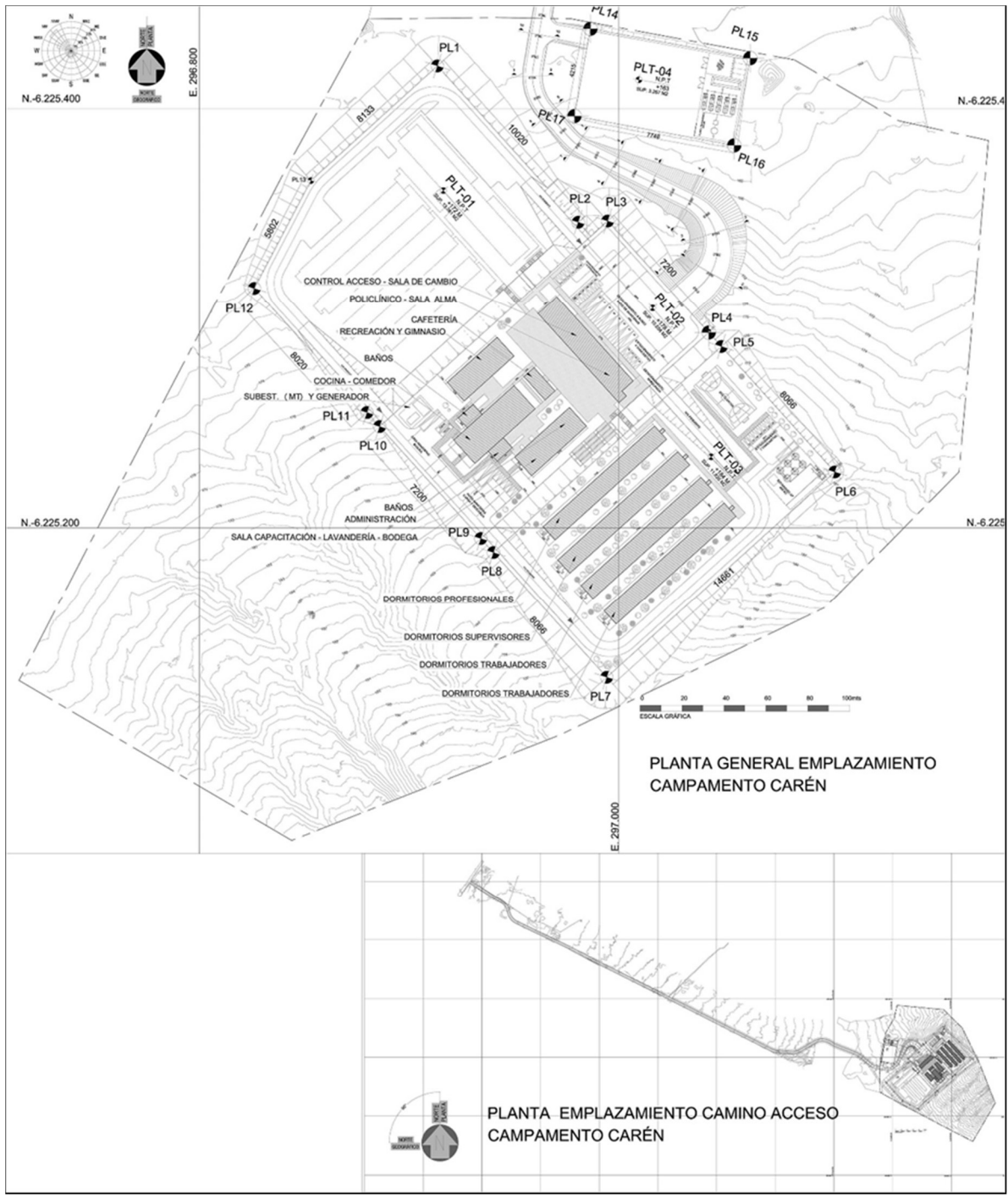
Figura 1: Layout Planta Nuevo Campamento Carén.
