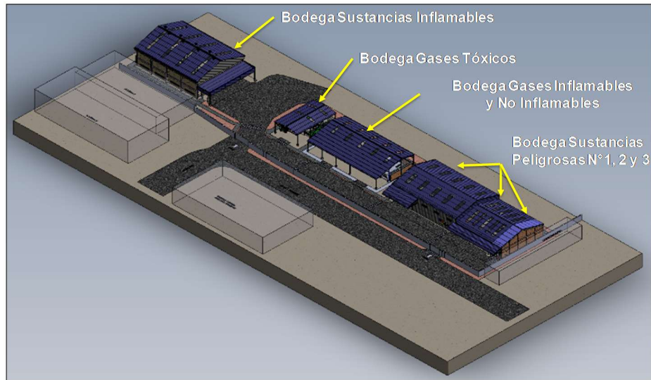
Figura N°1: Situación proyectada - Bodegas Centralizadas en "Patio de Fierros" de DVEN.
