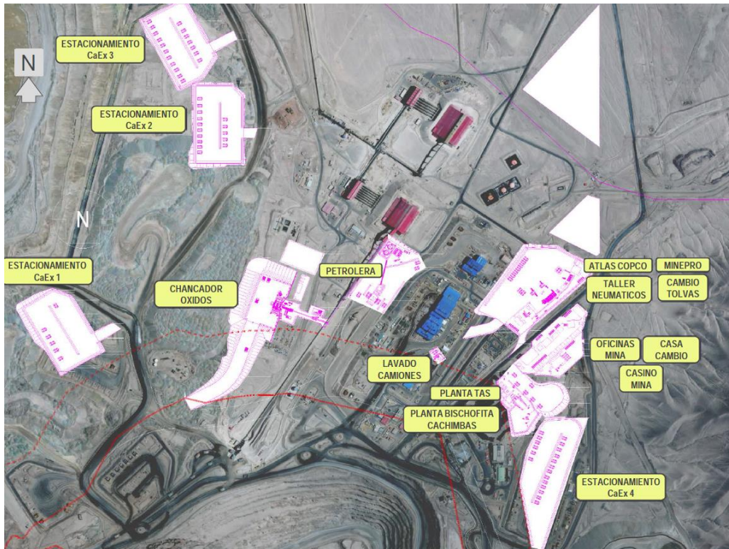
Figura 2-4 Ubicación propuesta de las nuevas Instalaciones
