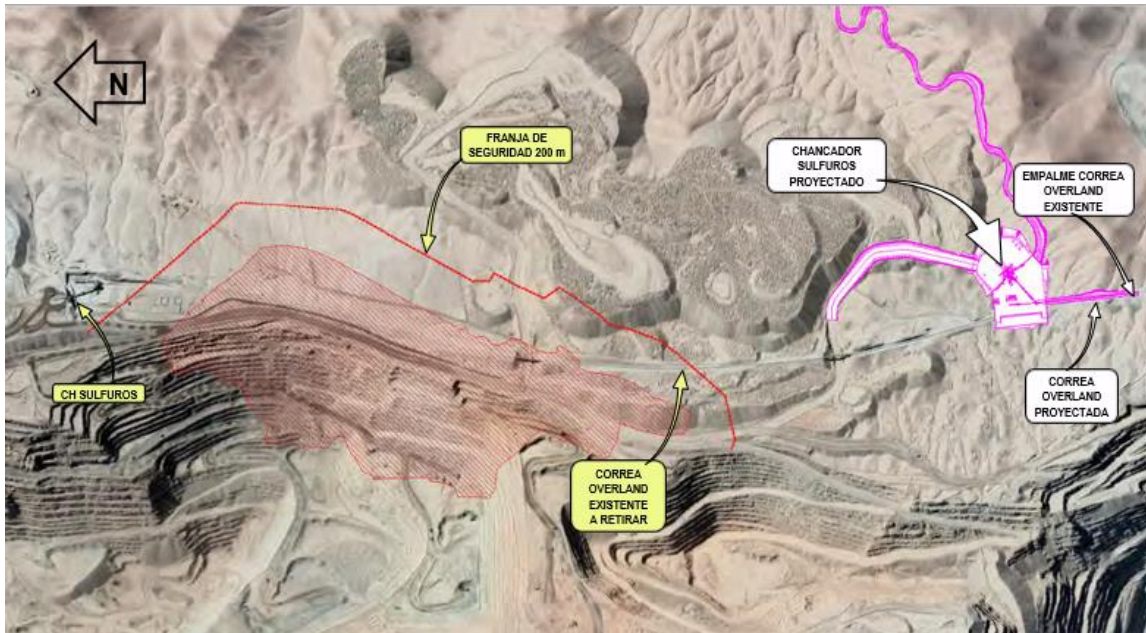
Figura 2-2. Instalaciones Nuevas y Afectadas desarrollo Zona Este
