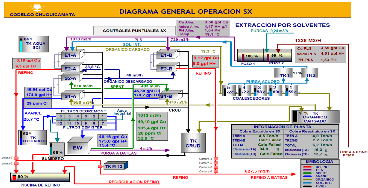
Esquema N° 4 Planta SX
