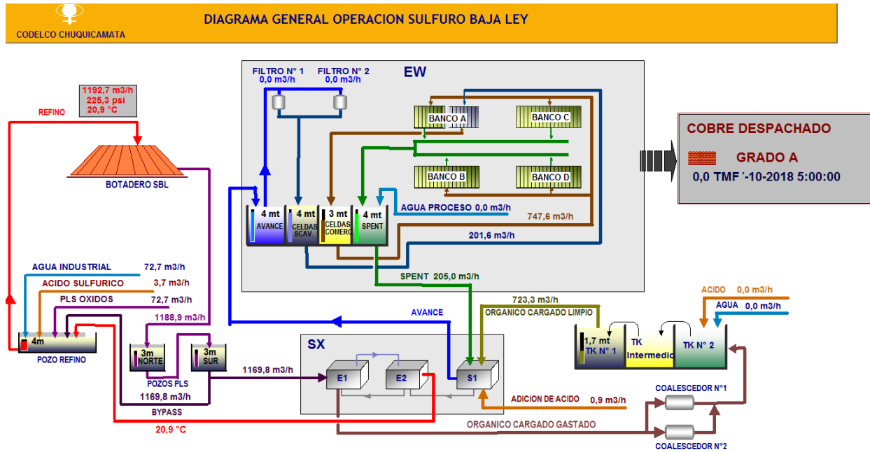
Esquema N° 4 Planta SBL
