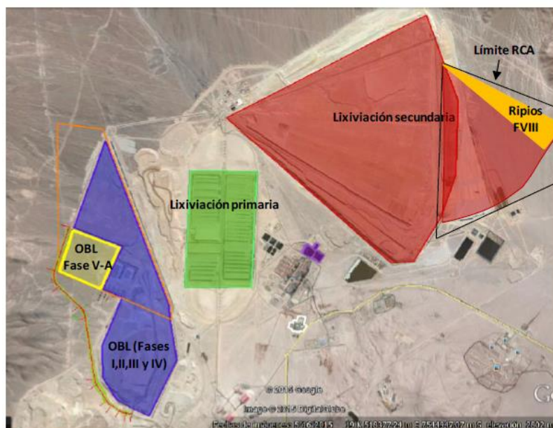
Figura 4.5: Ubicación Esquemática del Proyecto
