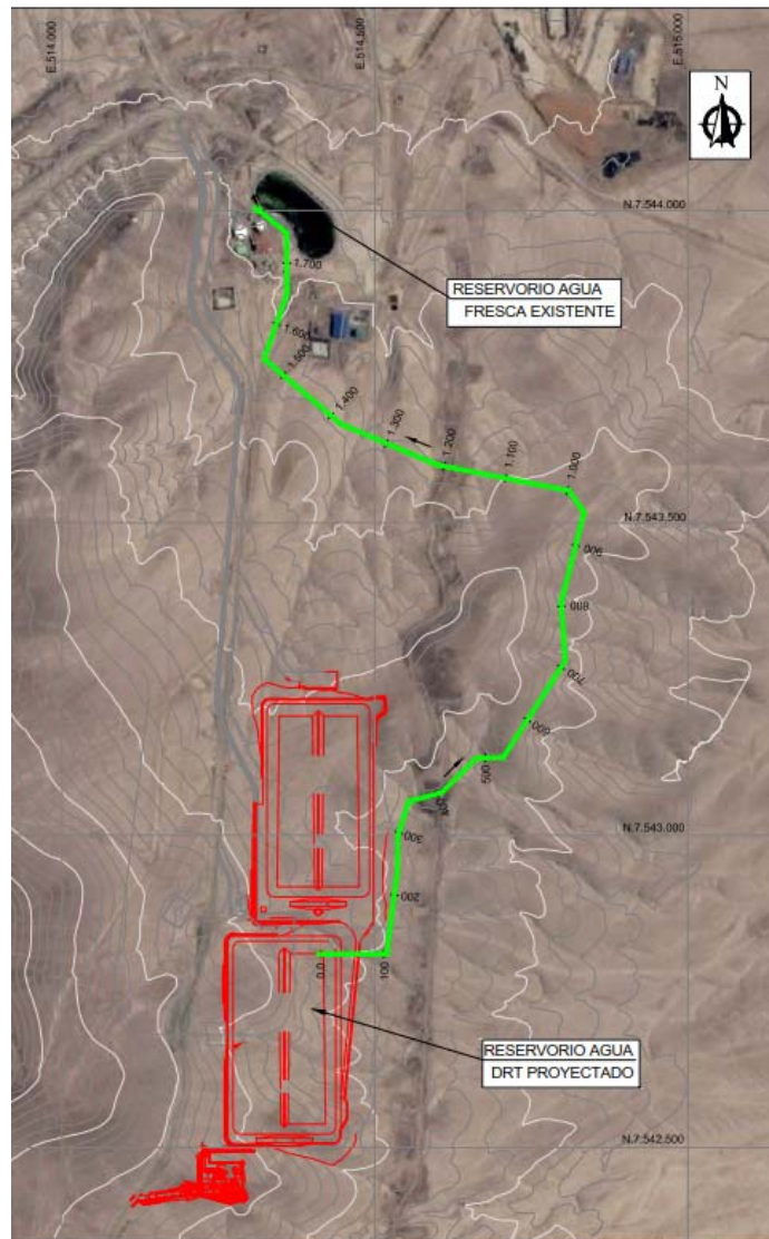
Figura 2-2. Trazado conducción reservorio industrial SADDN a reservorio Riñón existente en División Radomiro Tomic
