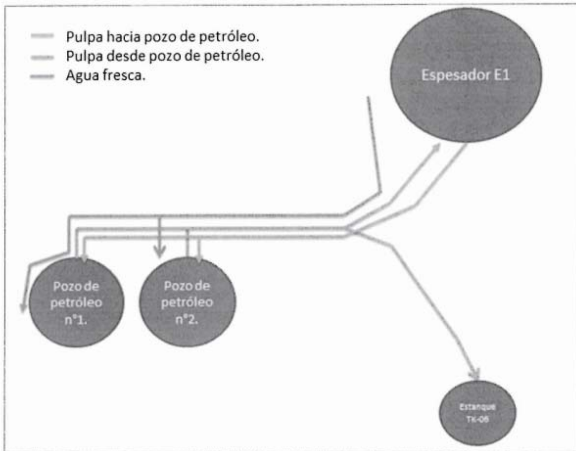
1.1 Diagrama esquemático de las actividades de tendido de redes para pulpa y agua.
