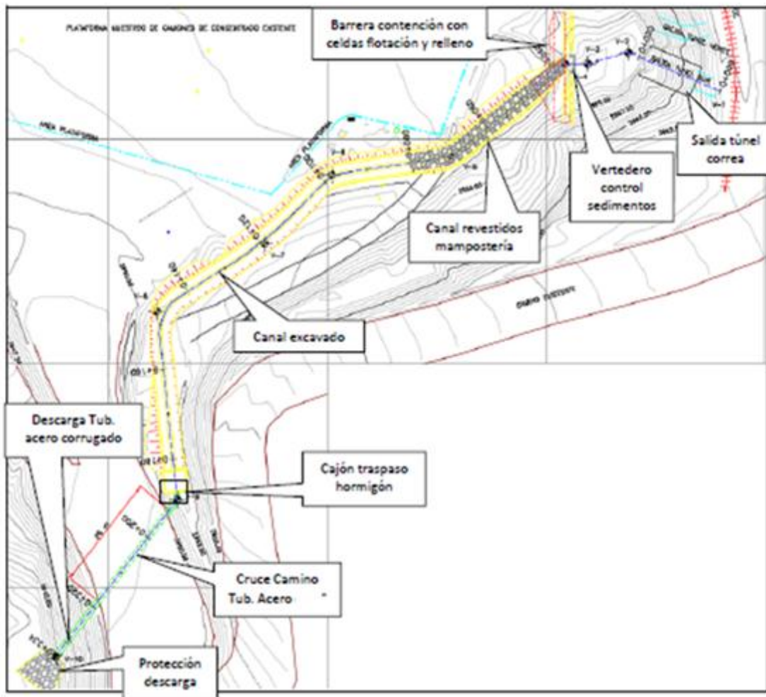
Figura N° 1: Planta esquemática de obras a ejecutar
