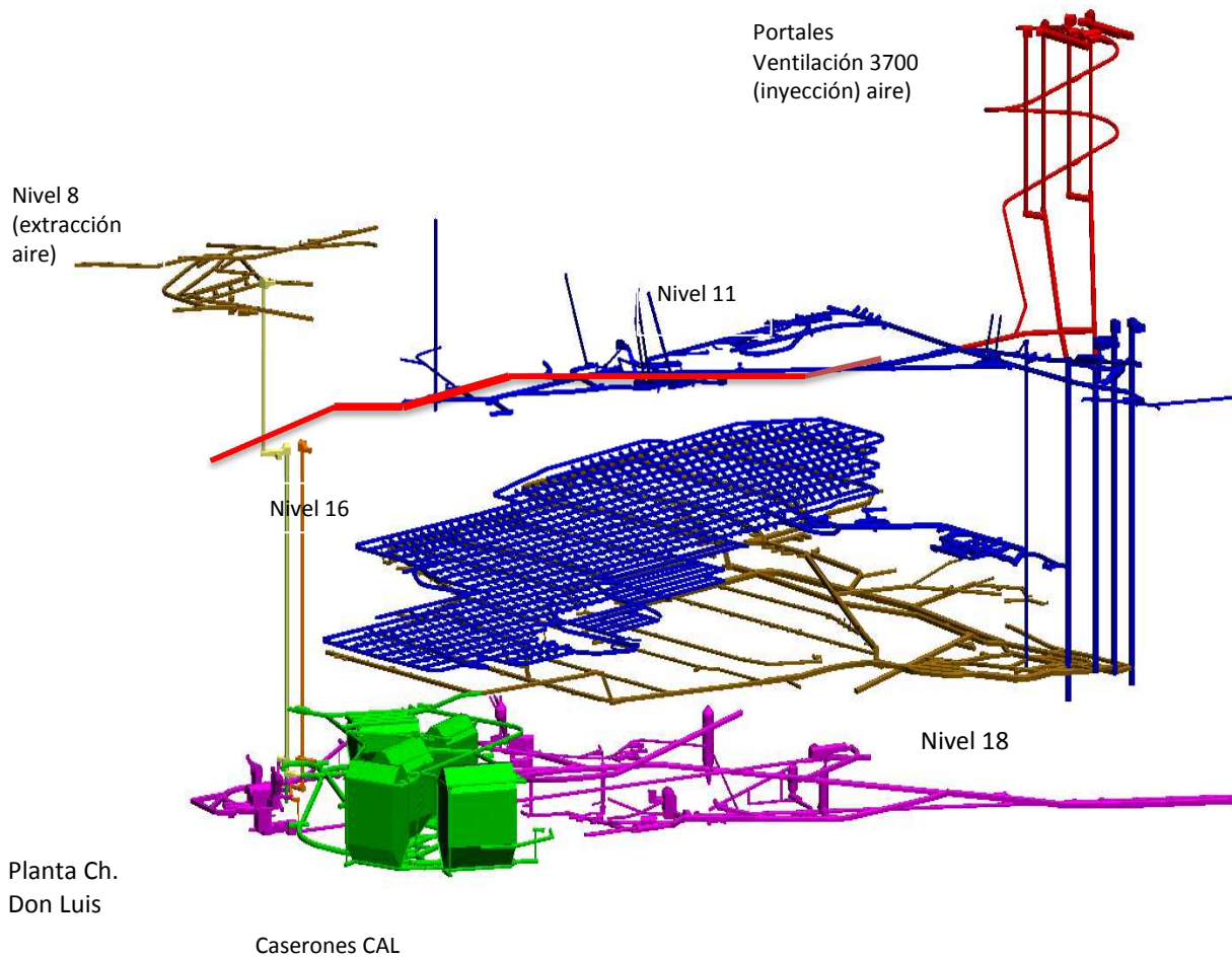
Plano 3D Mina Subterránea, con los sistemas de ventilación DAND
