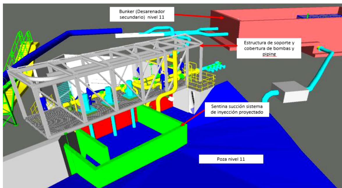
Figura 1: Esquema del Sistema de Inyección
