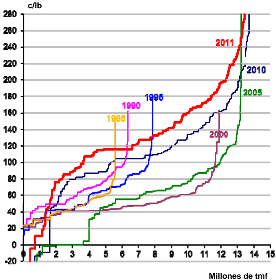
Oferta de Cobre de la Industria* Curva de Cash Cost (C1)
