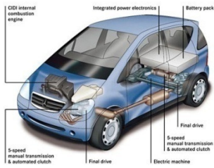
Autos Híbridos
