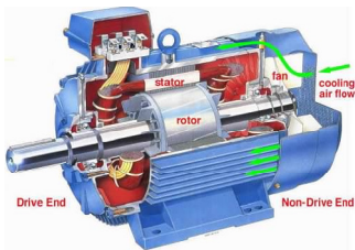
Motores de Alta Eficiencia
